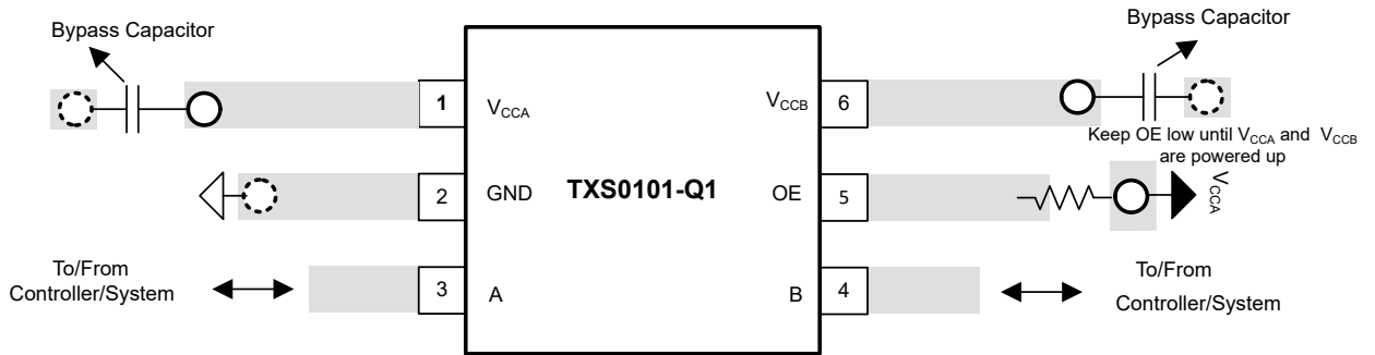
图 8-3. TXS0101-Q1 的典型布局
