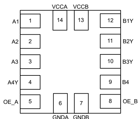
图 4-1. TXG4041-Q1 RUC 封装 14 引脚 X2QFN 顶视图
