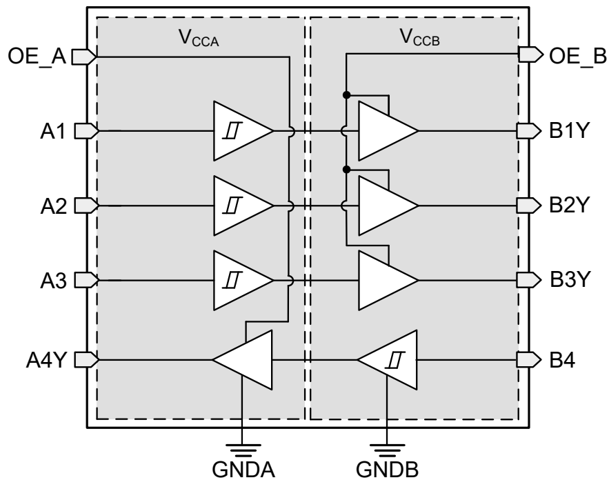
图 7-1. TXG1041 功能方框图
