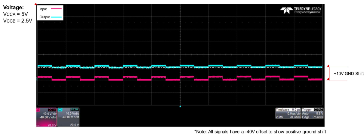
图 8-2. 显示了 5V 至 2.5V I/O 转换的 -10V (顶部) 和 +10V (底部) 接地漂移的波形
