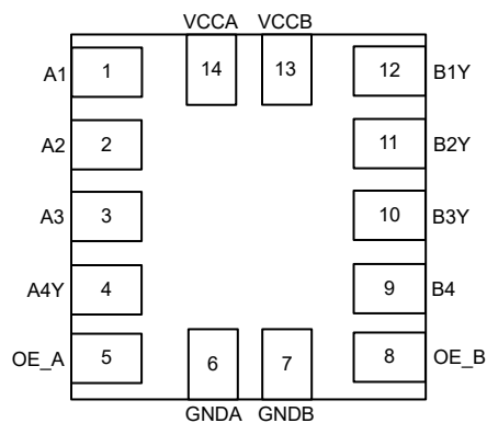
图 4-1. TXGx041RUC 封装 14 引脚 X2QFN 顶视图
