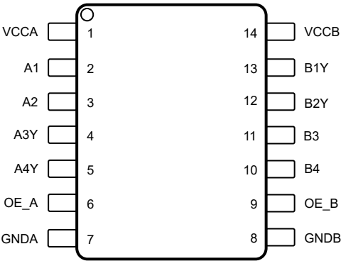
图 4-4. TXGx042DYY 14 引脚 SOT 顶视图
