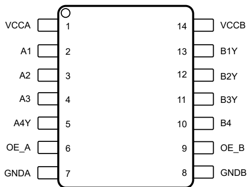
图 4-3. TXGx041DYY 14 引脚 SOT 顶视图
