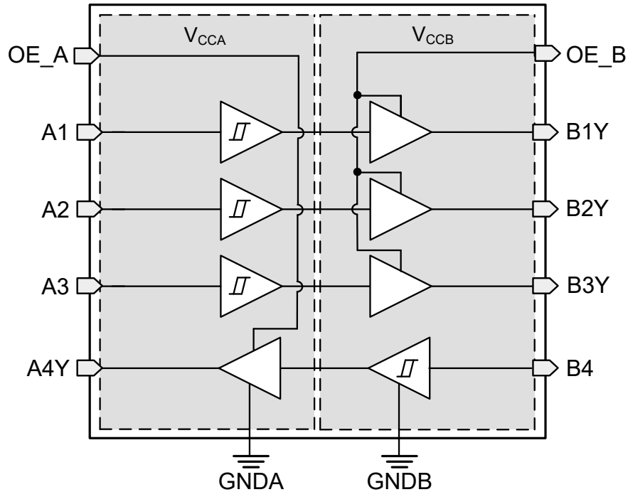
图 7-1. TXG1041-Q1 功能方框图
