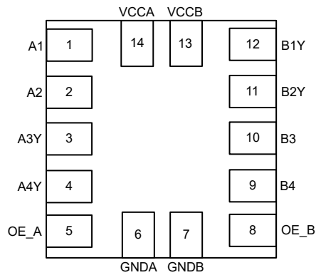
图 4-2. TXG1042-Q1 RUC 封装 14 引脚 X2QFN 顶视图
