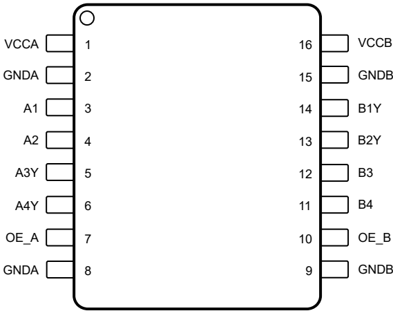
图 4-6. TXG1042-Q1 DBQ 16 引脚 QSOP 顶视图
