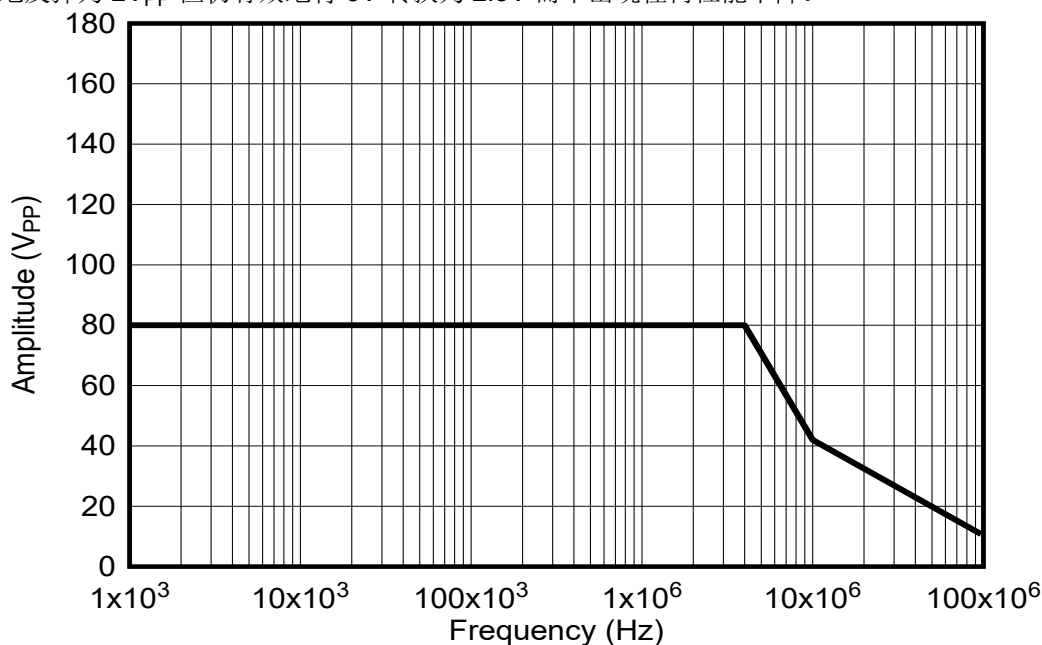
图 7-4. 交流噪声抑制图
