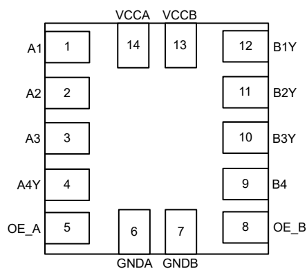
图 4-1. TXG1041-Q1 RUC 封装 14 引脚 X2QFN 顶视图
