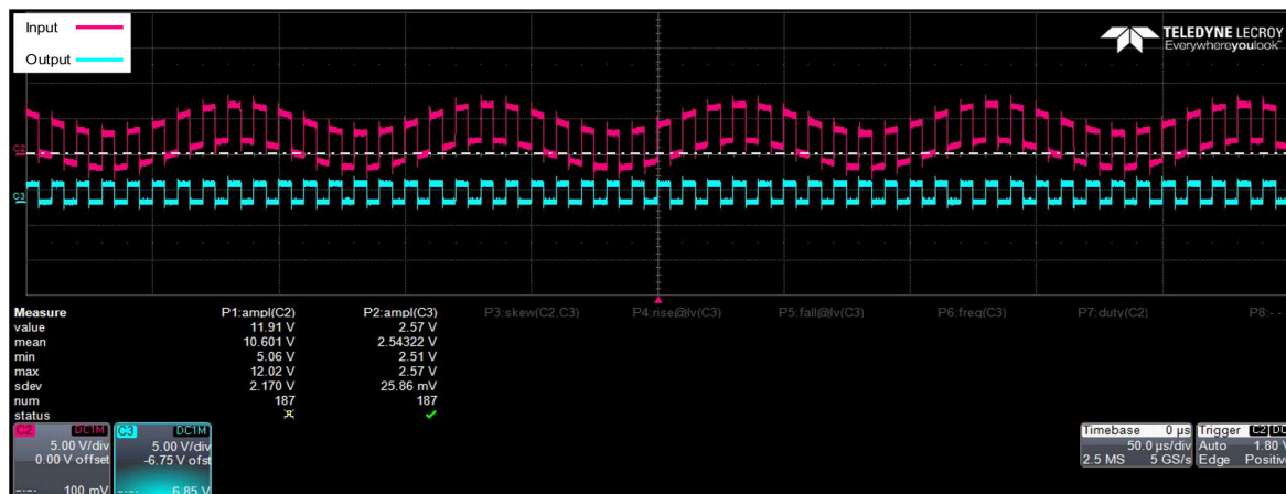
图 7-5. 显示了在交流接地噪声为 2V_{PP} (10kHz) 时 5V 至 2.5V I/O 转换的波形
