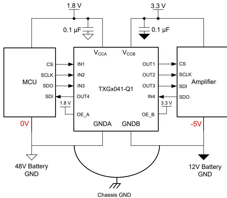
图 8-1. 汽车中的 TXG1041-Q1
