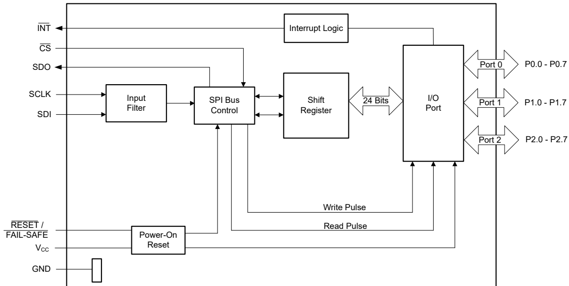
图 7-1. 逻辑图
