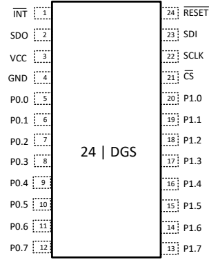
图 4-2. TXE8116-Q1 DGS (VSSOP) 封装，24 引脚 (顶视图)
