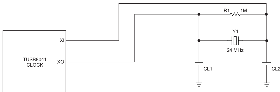
图 3. TUSB8041-Q1 Clock
