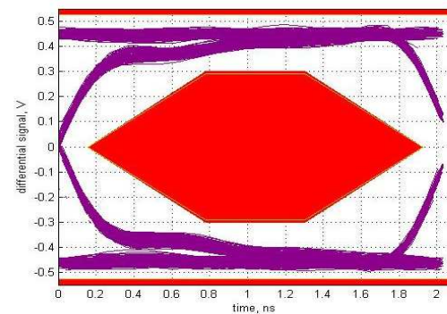
图 16. Downstream Port 3
