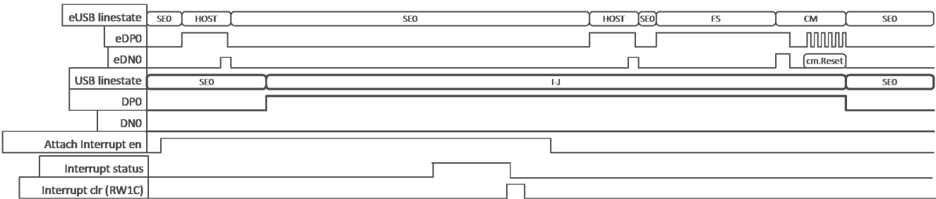
图 8-4. HS/FS 连接检测中断的时序图
