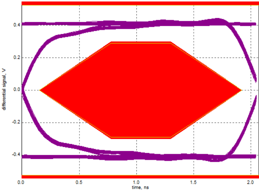
图 10-2. 典型 USB 2.0 高速眼图
