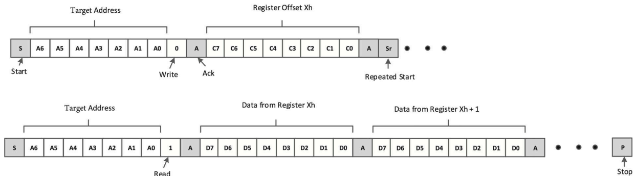
图 8-7. 使用重复启动的 I 2 C 读取
