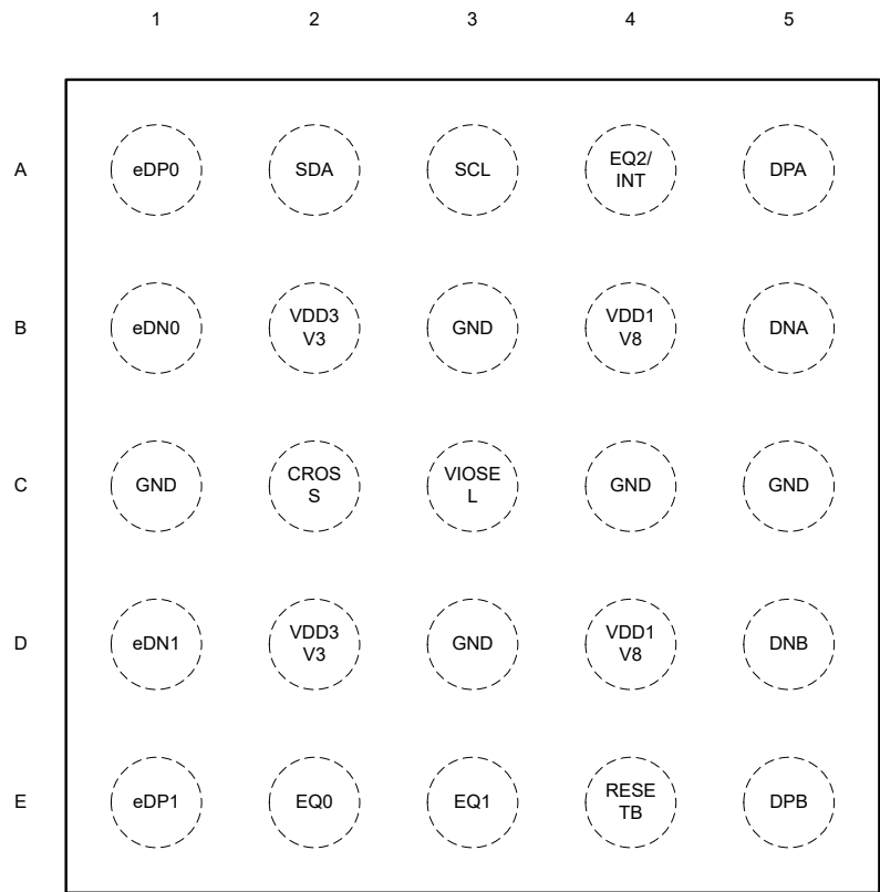
图 5-1. YCG 封装，25 引脚 DSBGA (俯视图)
