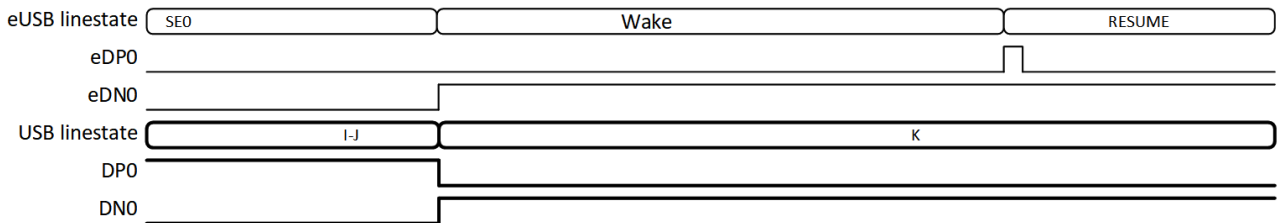
图 8-1. HS/FS 自动恢复的时序图
