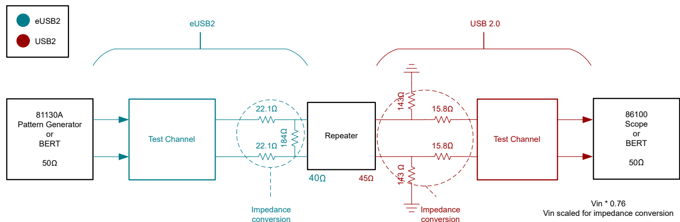
图 7-1. USB 2.0 TX 输出 (出口) 抖动、眼罩测试设置
