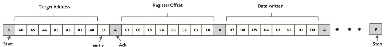
图 8-5. I 2 C 写入数据
