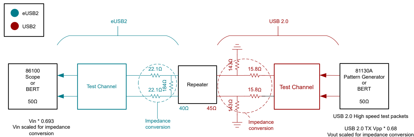
图 7-2. eUSB2 TX 输出 (入口) 抖动、眼罩测试设置
