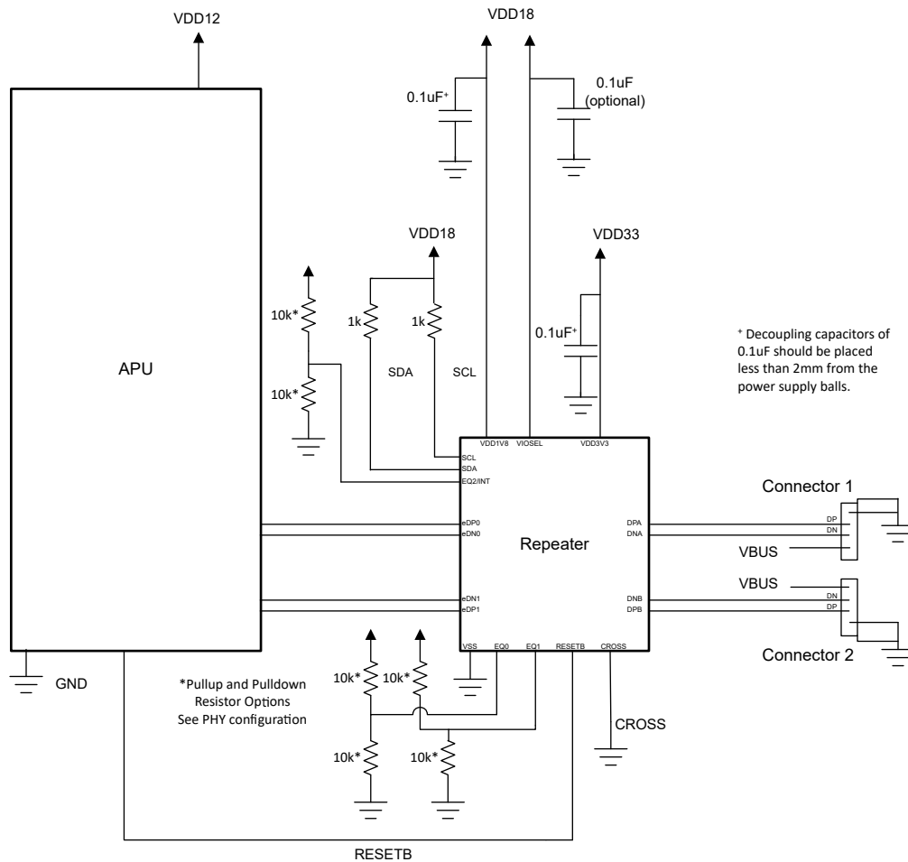
图 10-1. 使用 1.8V 和 I 2 C 的典型双端口系统实现
