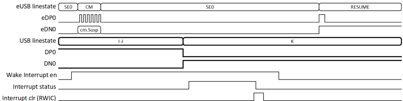
图 8-2. HS/FS 的唤醒中断时序图
