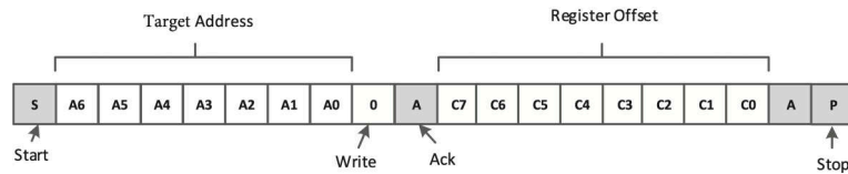
图 8-8. I 2 C 不带数据写入
