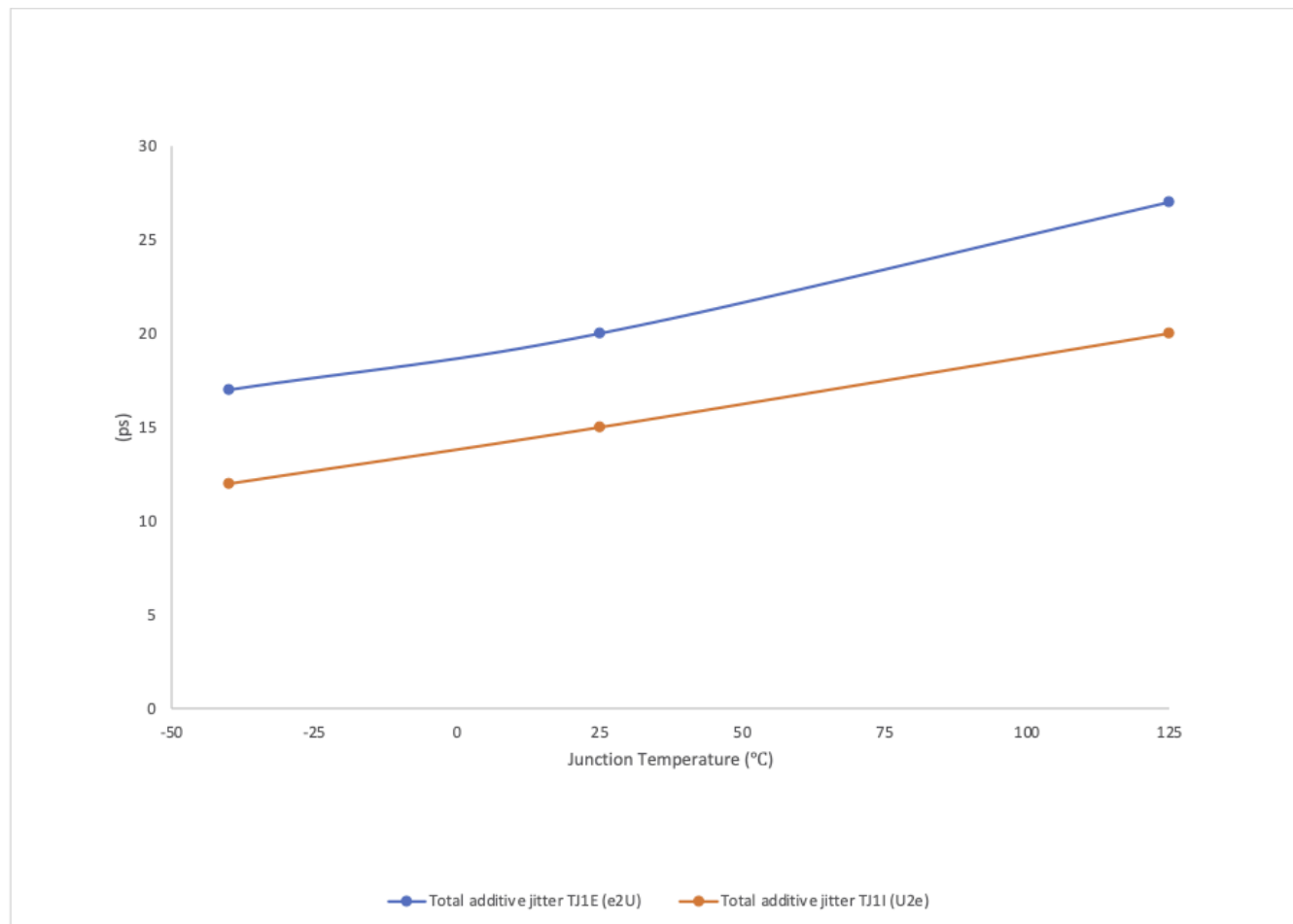
图 6-1. 总附加抖动 ( 典型值 )
