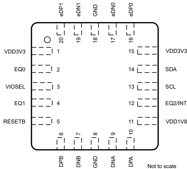
图 5-2. VBW 封装 20 引脚 WQFN (顶视图)
