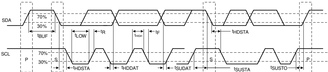
图 8-9. I 2 C 时序图
