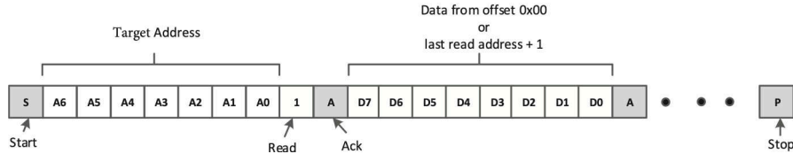
图 8-6. 不使用重复启动的 I 2 C 读取
