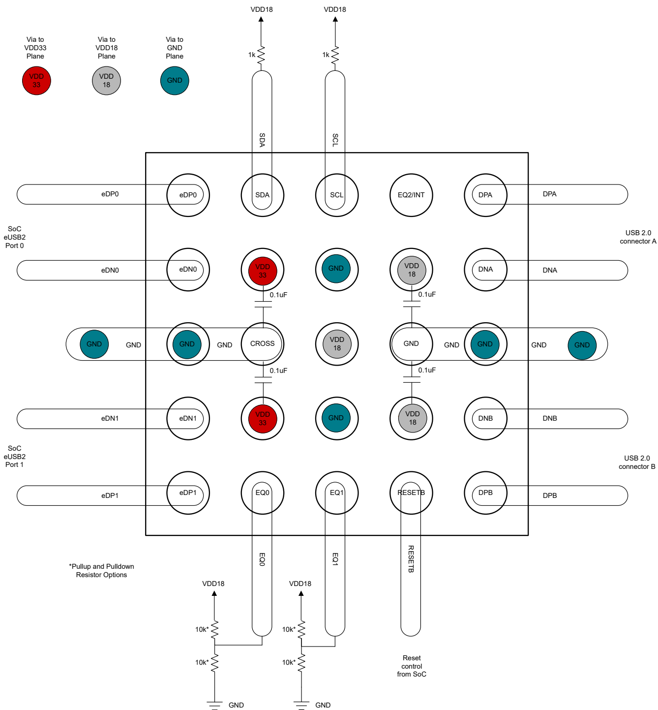
图 10-4. WCSP 的示例布局
