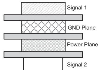
图 10-3. 四层板堆叠
