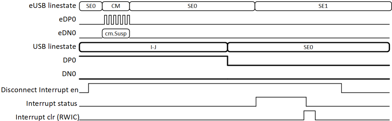
图 8-3. HS/FS 断开中断的时序图
