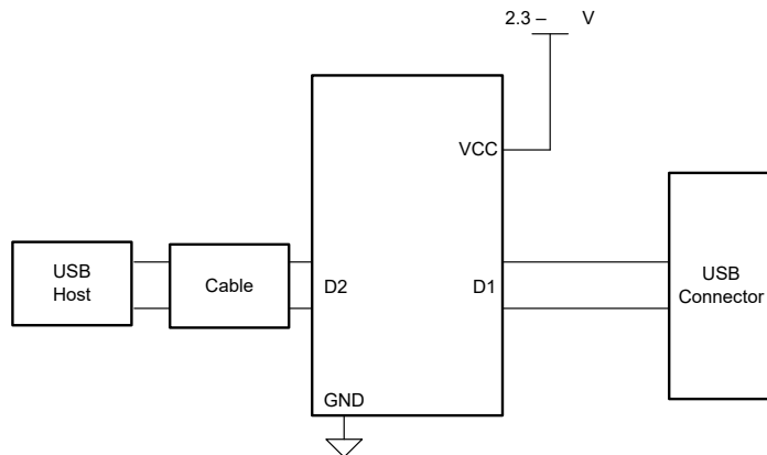
简化原理图
