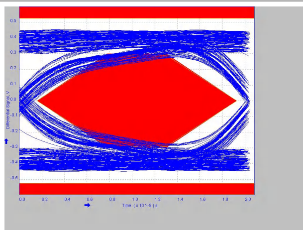
图 8-5. 5 Meter Without TUSB211A
