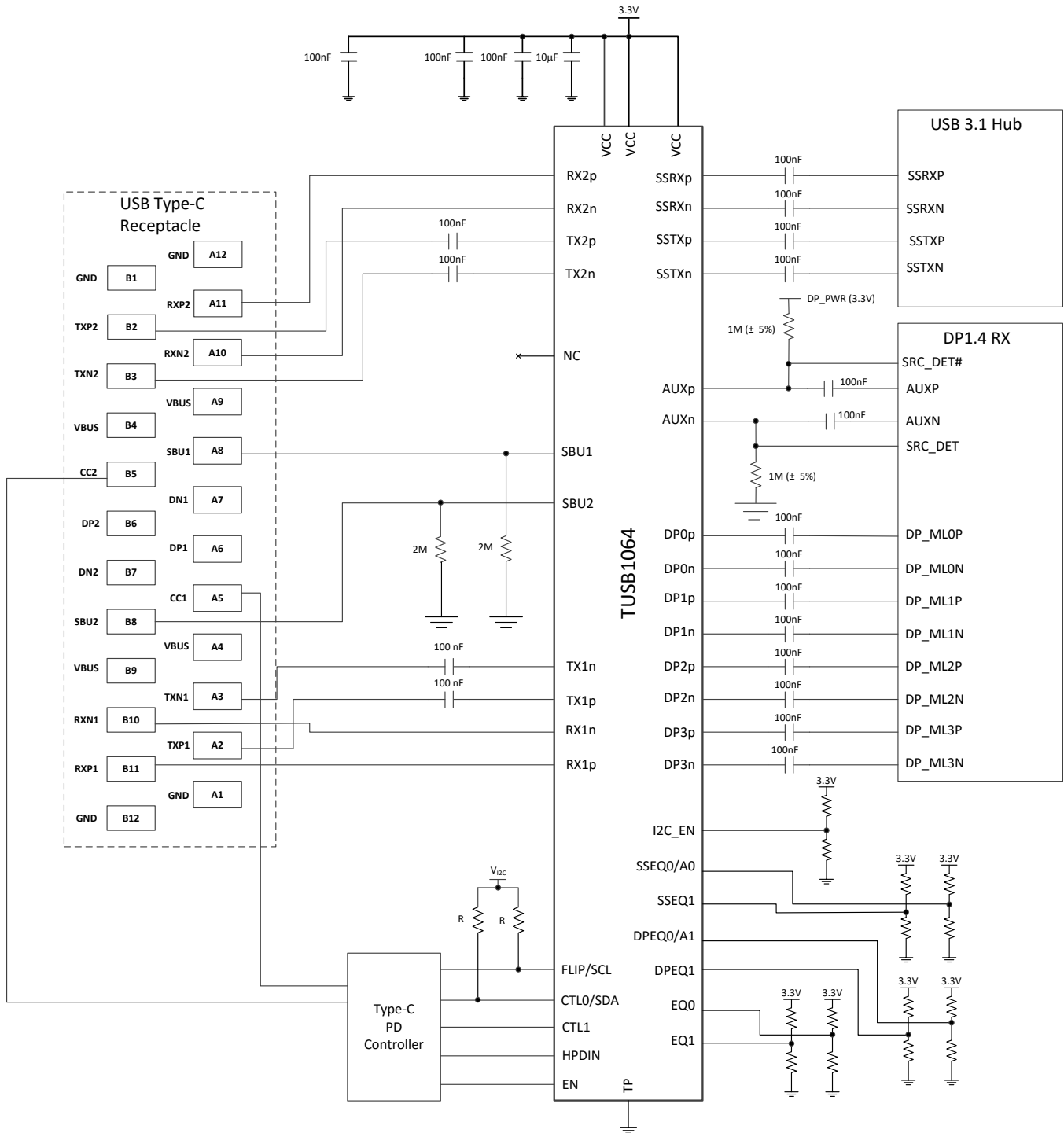
图 27. Application Circuit
