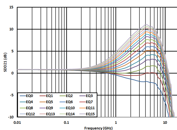
图 2. USB RX (DFP) EQ Settings Curves
