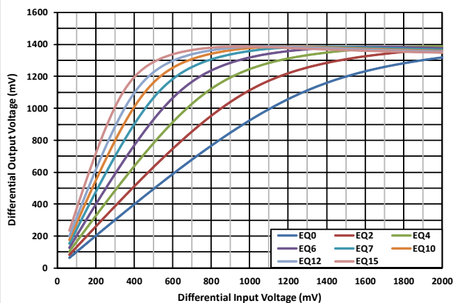
图 2. USB RX (DFP) EQ Settings Curves
