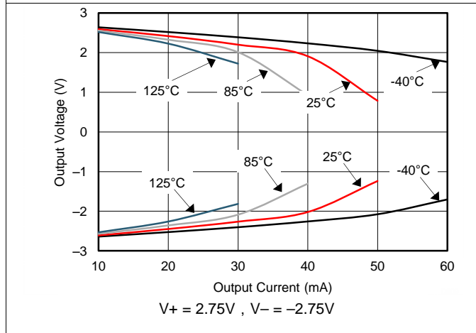
图 9. 输出电压摆幅与输出电流间的关系
