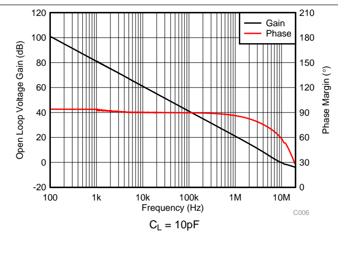
图 6. 开环增益和相位与频率间的关系
