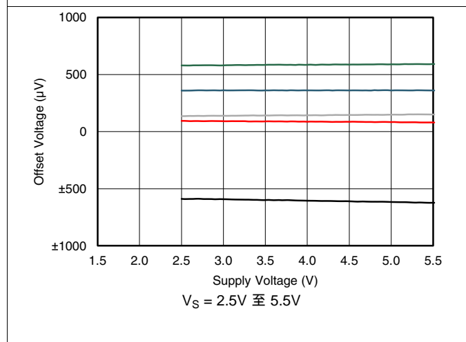
图 5. 失调电压与电源间的关系
