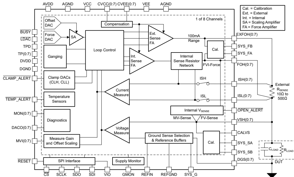
方框图
