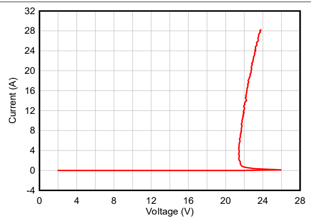
图 5-2. 正 TLP 曲线 - TSD15-Q1
