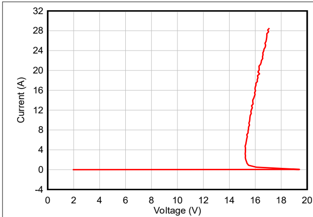
图 5-1. 正 TLP 曲线 - TSD12-Q1
