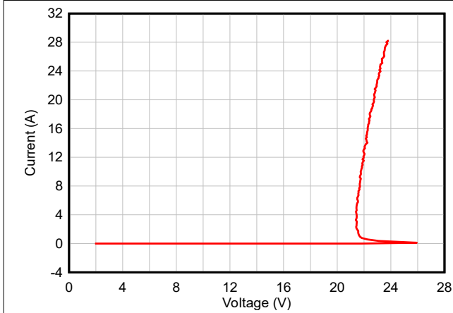
图 5-3. 正 TLP 曲线 - TSD18-Q1
