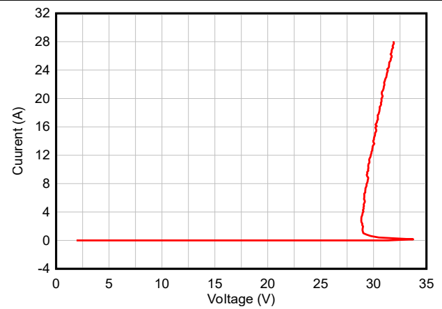
图 5-4. 正 TLP 曲线 - TSD24-Q1
