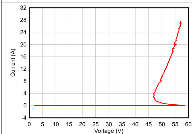
图 5-5. 正 TLP 曲线 - TSD36-Q1
