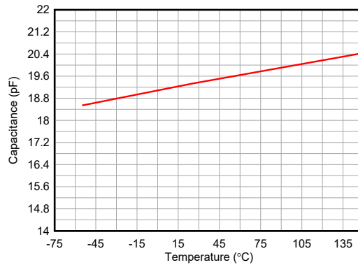
图 5-11. 温度与电容间的关系 - TSD05
