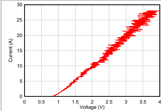
图 5-3. 负 TLP 曲线 - TSD05
