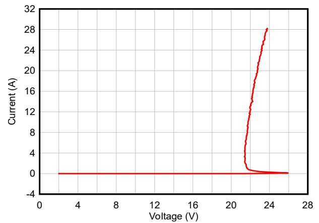
图 5-6. 正 TLP 曲线 - TSD18
