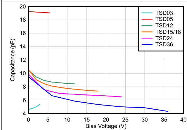
图 5-9. 电容与偏置电压之间的关系
