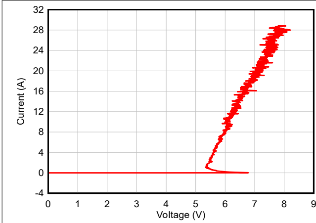
图 5-1. 正 TLP 曲线 - TSD03
