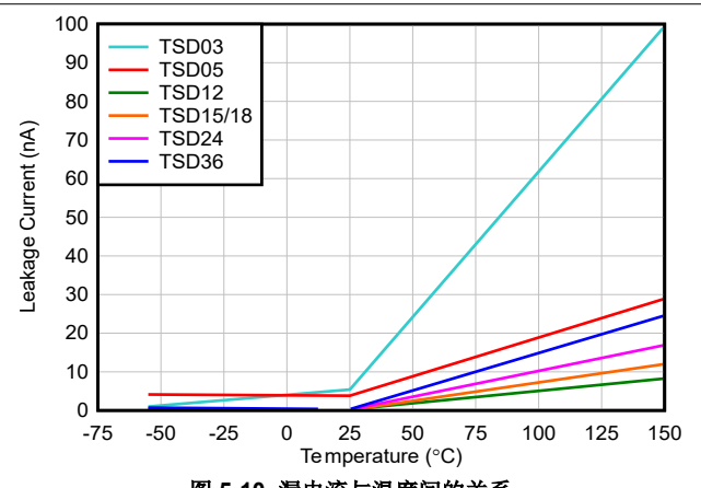
图 5-10. 漏电流与温度间的关系
