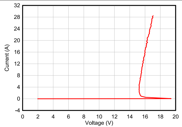
图 5-4. 正 TLP 曲线 - TSD12
