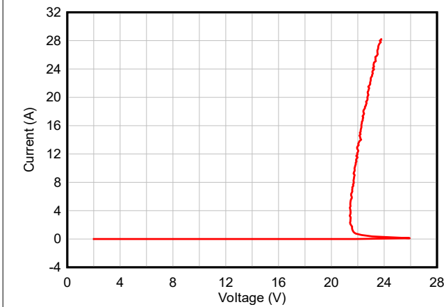
图 5-5. 正 TLP 曲线 - TSD15
