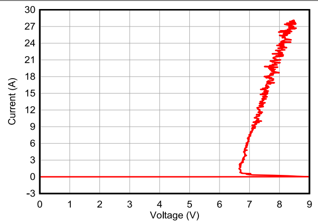
图 5-2. 正 TLP 曲线 - TSD05
