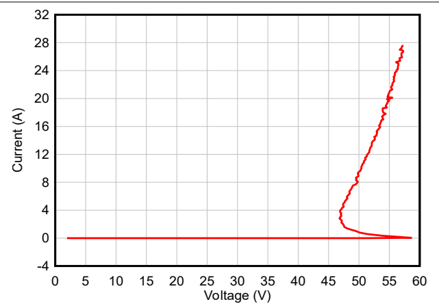
图 5-8. 正 TLP 曲线 - TSD36
