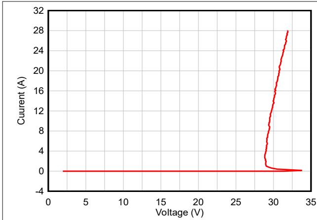
图 5-7. 正 TLP 曲线 - TSD24
