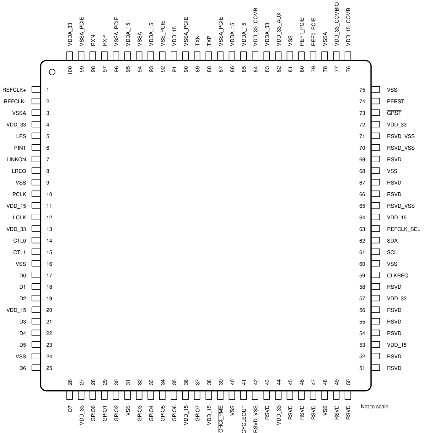
图 5-1. PZT Package 100-Pin QFP Top View
