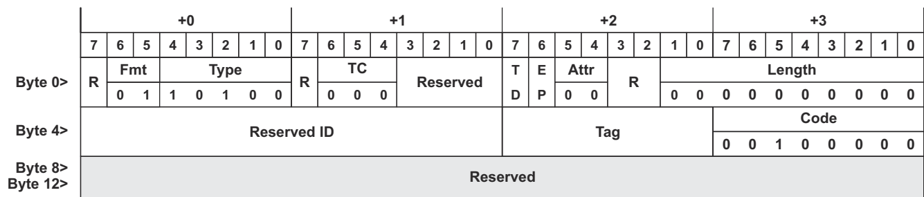
图 10-4. PCIe Assert_INTA Message
