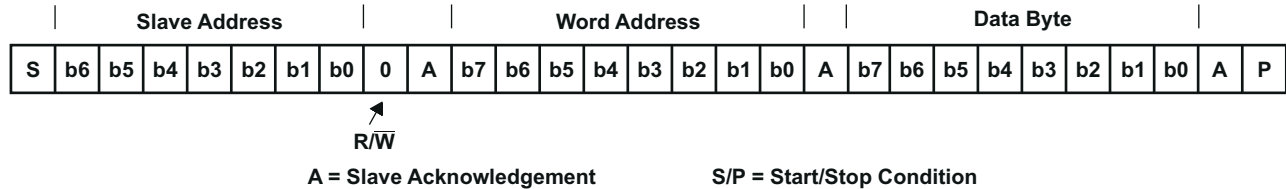
图 10-9. Serial-Bus Protocol Byte Write
