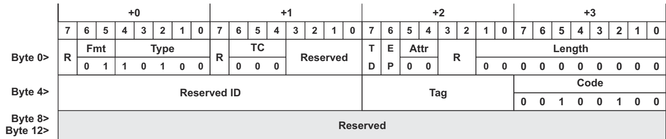
图 10-5. PCIe Deassert_INTX Message
