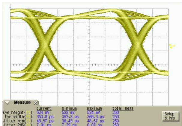
图 8-1. TSB82AF15-EP Eye Diagram
