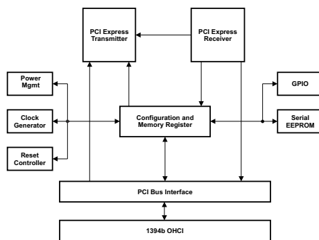
简化版方框图
