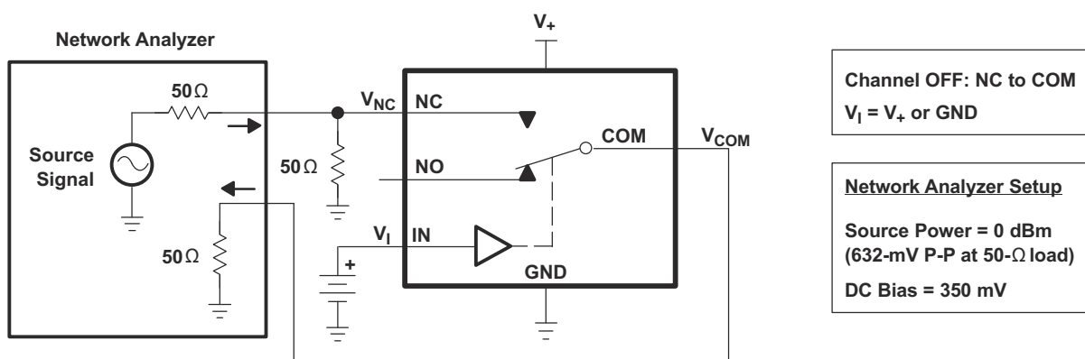
图 6-8. 关断隔离 ( O_{iso} )
