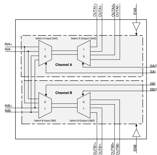
功能方框图
