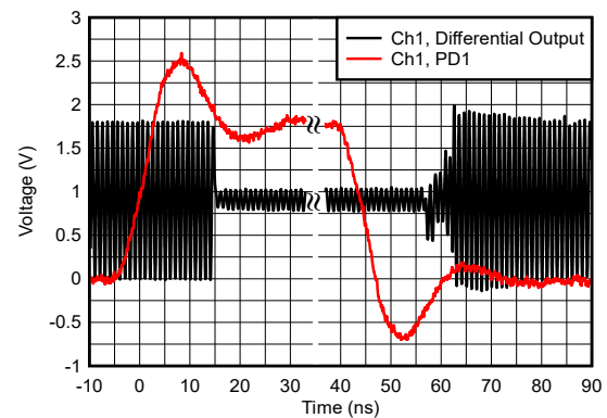
图 6-118. 阶跃响应
