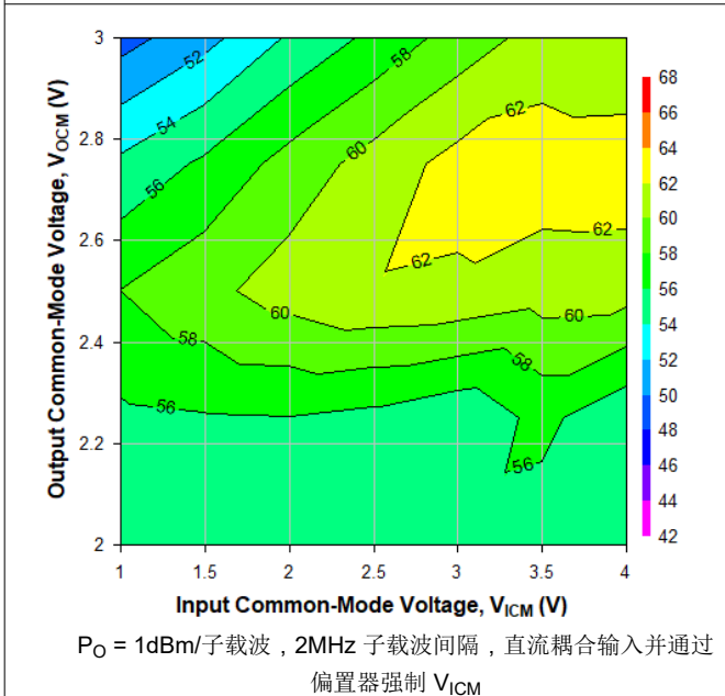
图 6-51. 2GHz 时不同 V_{ICM} 和 V_{OCM} 条件下的 OIP2, Ch1
