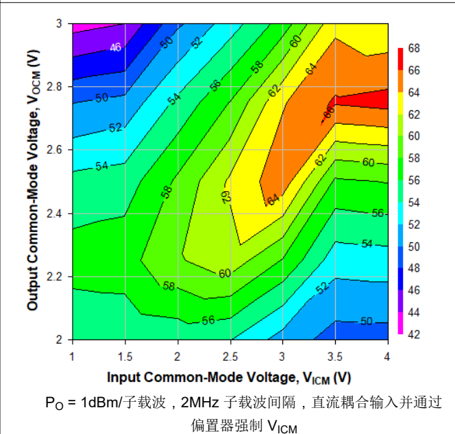
图 6-52. 2GHz 时不同 V_{ICM} 和 V_{OCM} 条件下的 OIP2, Ch2
