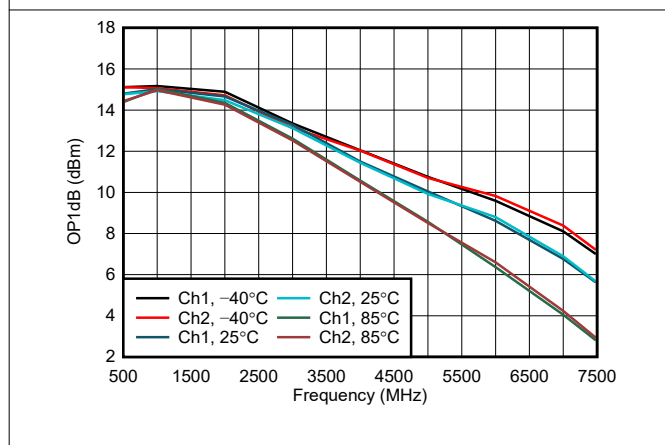
图 6-114. 整个温度范围内的 OP1dB
