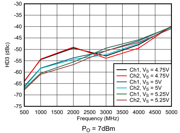
图 6-38. 整个电源电压范围内的 HD3
