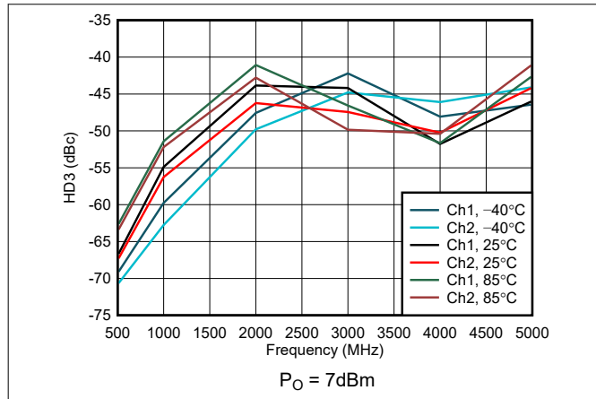
图 6-110. 整个温度范围内的 HD3
