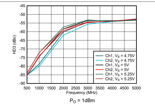
图 6-113. 整个电源电压范围内的 HD3
