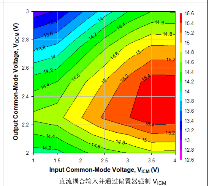
图 6-56. 2GHz 时不同 V_{ICM} 和 V_{OCM} 条件下的 OP1dB，Ch2
