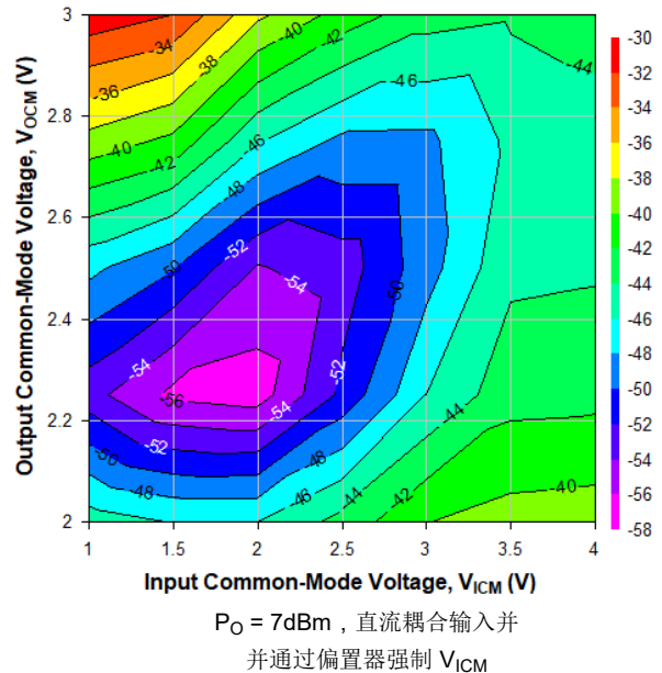
图 6-64. 2GHz 时不同 V_{\text{ICM}} 和 V_{\text{OCM}} 条件下的 HD3, Ch2
