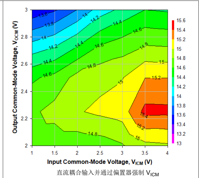
图 6-54. 500MHz 时不同 V_{ICM} 和 V_{OCM} 条件下的 OP1dB，Ch2
