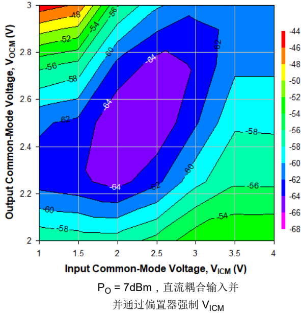
图 6-61. 500MHz 时不同 V_{\text{ICM}} 和 V_{\text{OCM}} 条件下的 HD3, Ch1
