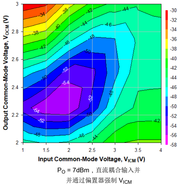
图 6-63. 2GHz 时不同 V_{\text{ICM}} 和 V_{\text{OCM}} 条件下的 HD3, Ch1
