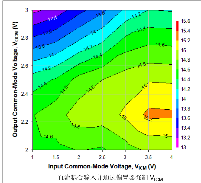
图 6-53. 500MHz 时不同 V_{ICM} 和 V_{OCM} 条件下的 OP1dB，Ch1
