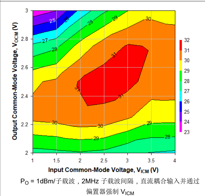
图 6-48. 2GHz 时不同 V_{ICM} 和 V_{OCM} 条件下的 OIP3, Ch2
