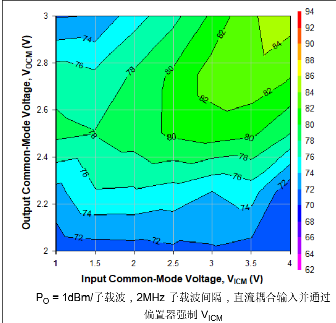
图 6-49. 500MHz 时不同 V_{ICM} 和 V_{OCM} 条件下的 OIP2, Ch1
