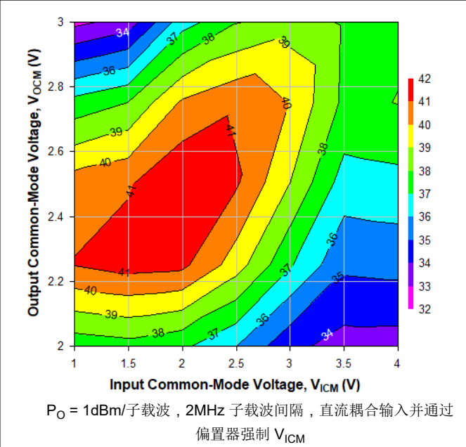
图 6-46. 500MHz 时不同 V_{ICM} 和 V_{OCM} 条件下的 OIP3, Ch2
