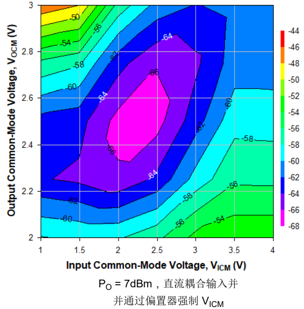
图 6-62. 500MHz 时不同 V_{\text{ICM}} 和 V_{\text{OCM}} 条件下的 HD3, Ch2
