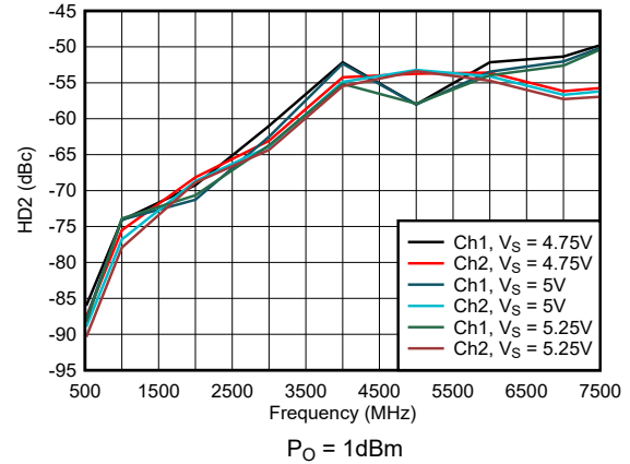
图 6-36. 整个电源电压范围内的 HD2
