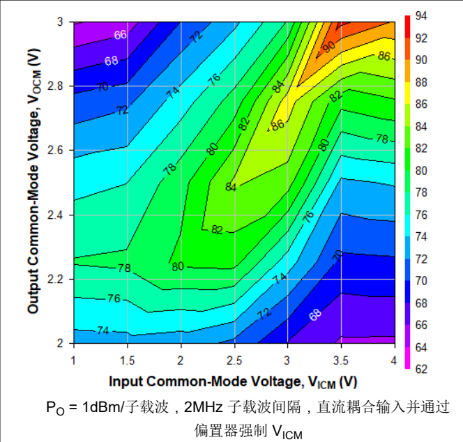
图 6-50. 500MHz 时不同 V_{ICM} 和 V_{OCM} 条件下的 OIP2, Ch2
