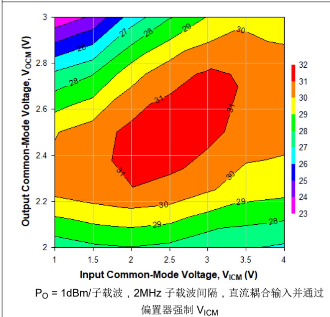
图 6-47. 2GHz 时不同 V_{ICM} 和 V_{OCM} 条件下的 OIP3, Ch1
