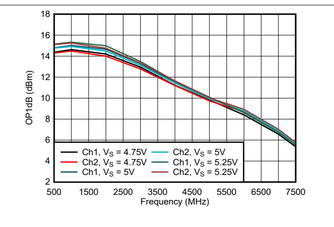
图 6-115. 整个电源电压范围内的 OP1dB
