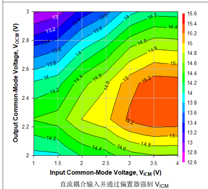
图 6-55. 2GHz 时不同 V_{ICM} 和 V_{OCM} 条件下的 OP1dB，Ch1
