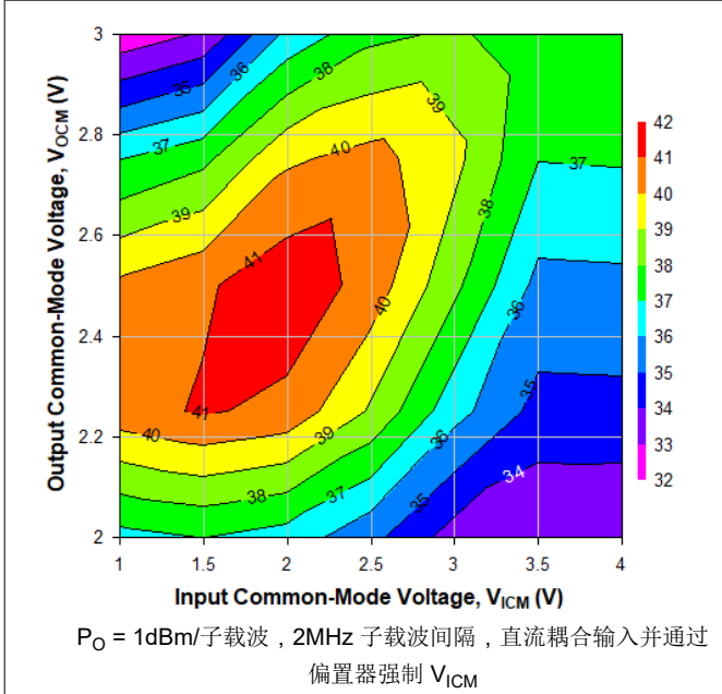
图 6-45. 500MHz 时不同 V_{ICM} 和 V_{OCM} 条件下的 OIP3, Ch1
