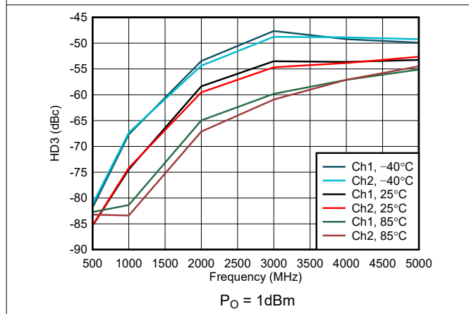
图 6-112. 整个温度范围内的 HD3
