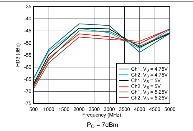
图 6-111. 整个电源电压范围内的 HD3
