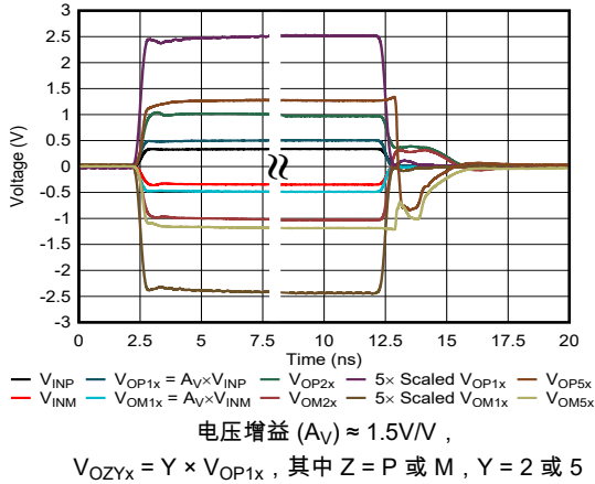
图 6-33. 过载恢复响应和时序
