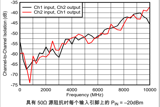
图 6-32. 通道间隔离
