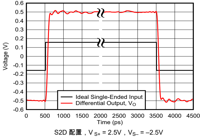
图 6-31. 阶跃响应
