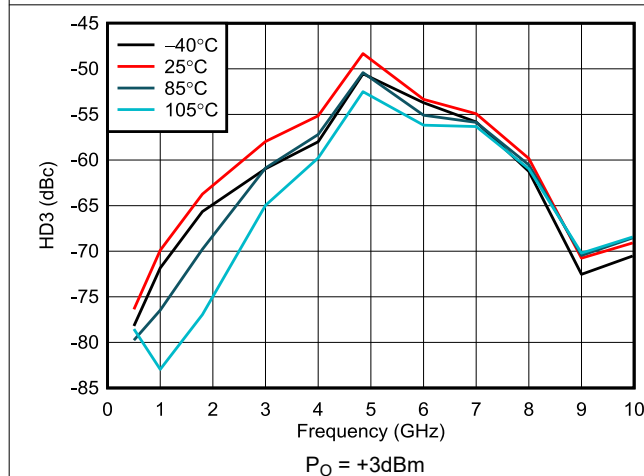
图 5-23. 整个温度范围内的 HD3
