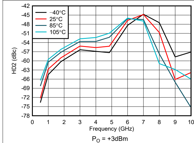
图 5-21. 整个温度范围内的 HD2
