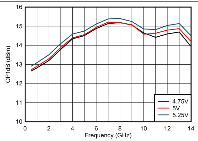
图 5-26. 整个 V_{DD} 范围内的输出 P1dB
