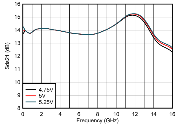
图 5-2. 整个 V_{DD} 范围内的功率增益
