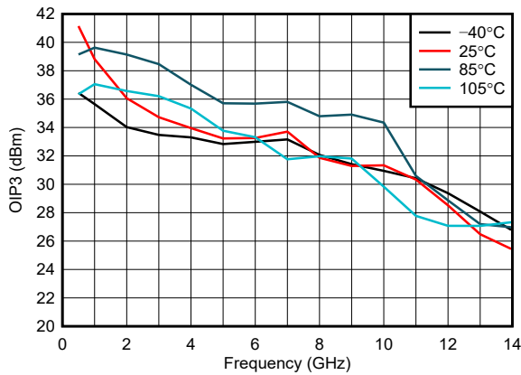
图 5-7. 整个温度范围内的 OIP3
