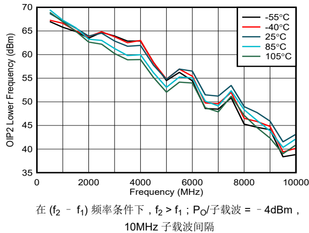
图 5-13. 整个温度范围内的 OIP2 更低
