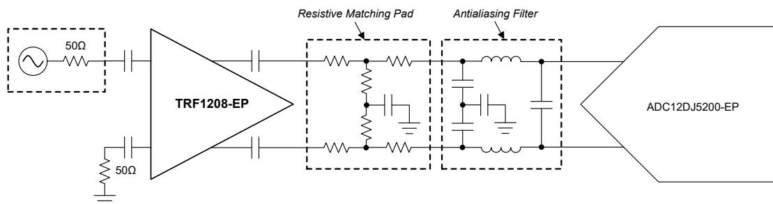
图 7-1. 与 ADC12DJ5200-EP 连接
