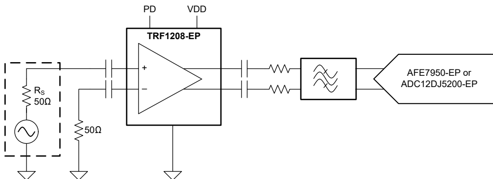
驱动高速 ADC 的 TRF1208-EP
