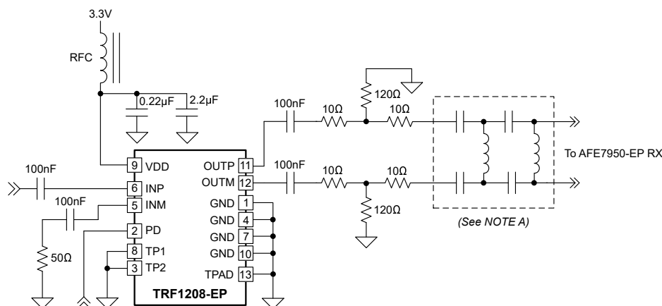
图 7-2. 与 AFE7950-EP 连接
