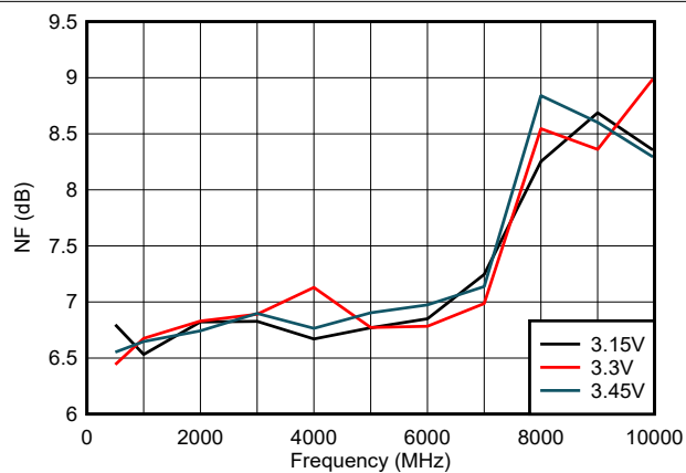
图 5-30. 整个 V_{DD} 范围内的 NF
