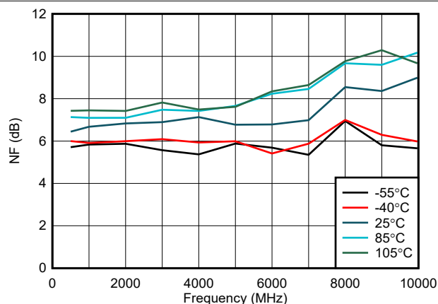
图 5-29. 整个温度范围内的 NF
