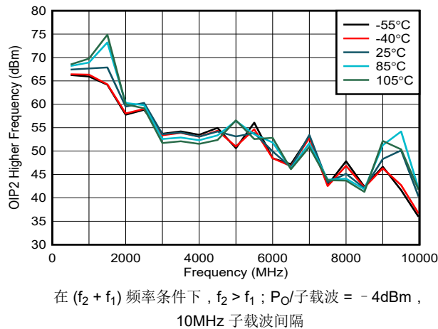
图 5-15. 整个温度范围内的 OIP2 更高
