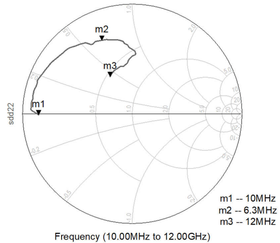
图 5-40. 差分 S22
