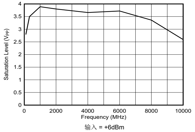
图 5-36. 饱和电压 (差分)
