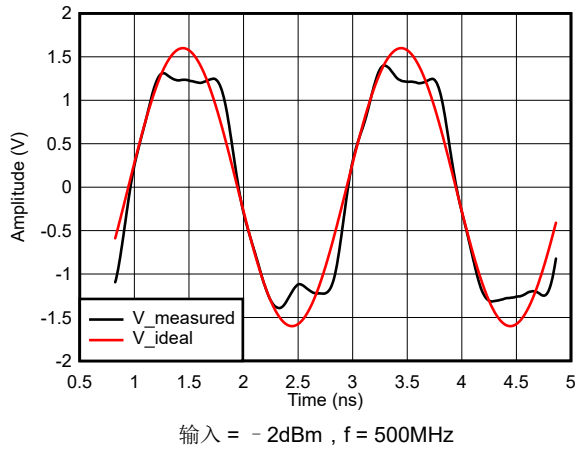
图 5-35. 过驱恢复
