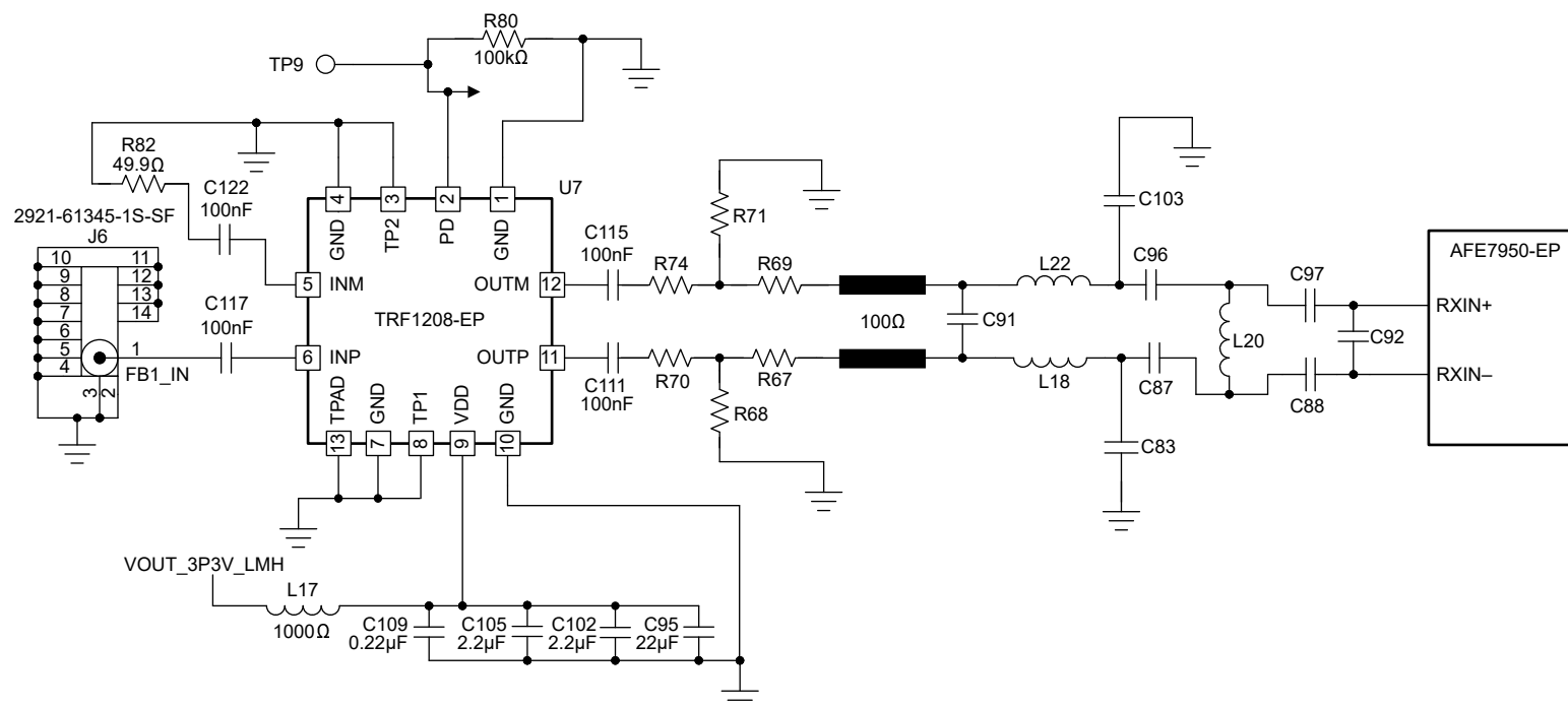
图 7-4. TRF1208-EP 在采用 AFE7950-EP 的接收链中
