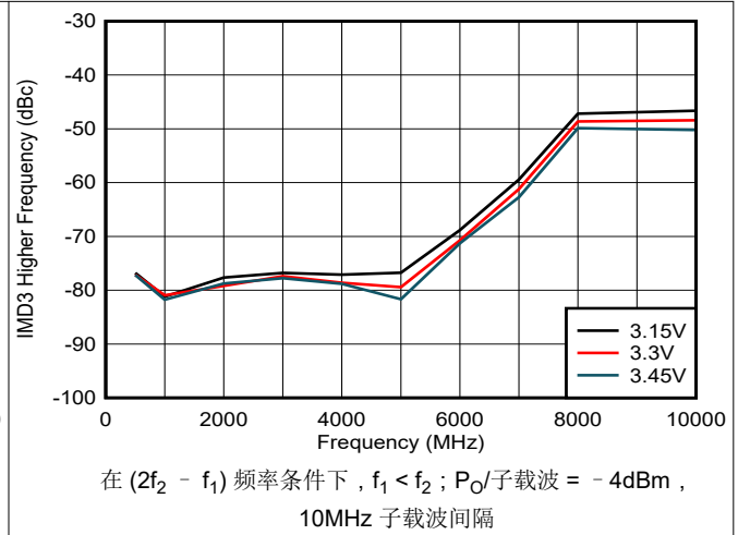
图 5-12. 整个 V_{DD} 范围内的 IMD3 更高
