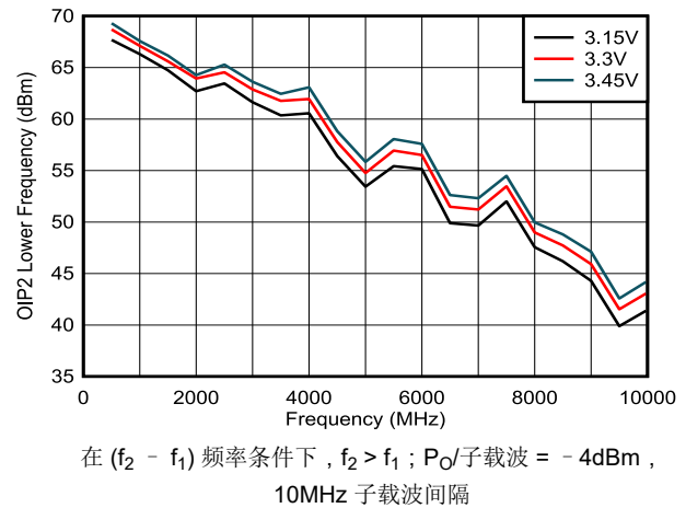
图 5-14. 整个 V_{DD} 范围内的 OIP2 更低
