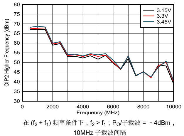
图 5-16. 整个 V_{DD} 范围内的 OIP2 更高
