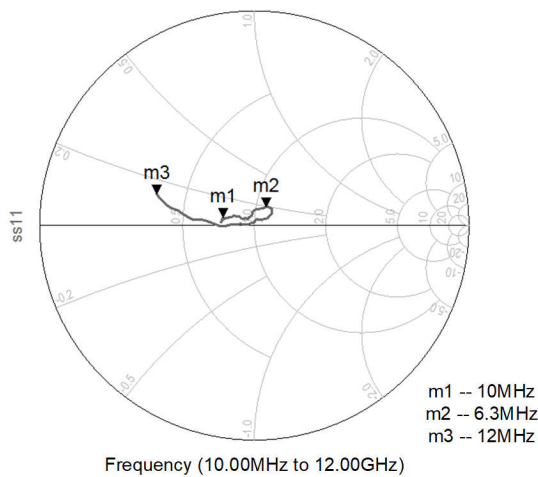
图 5-39. 单端 S11
