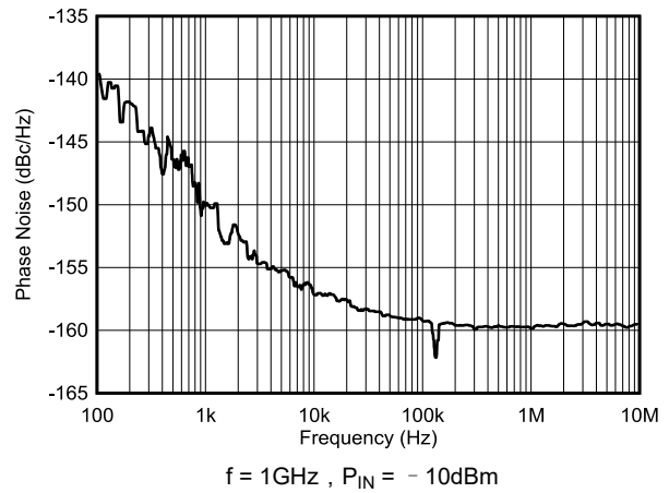
图 5-38. 附加 (残留) 相位噪声
