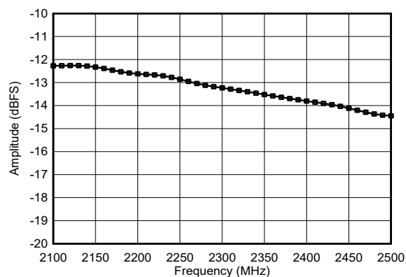
图 7-5. 带内输出响应
