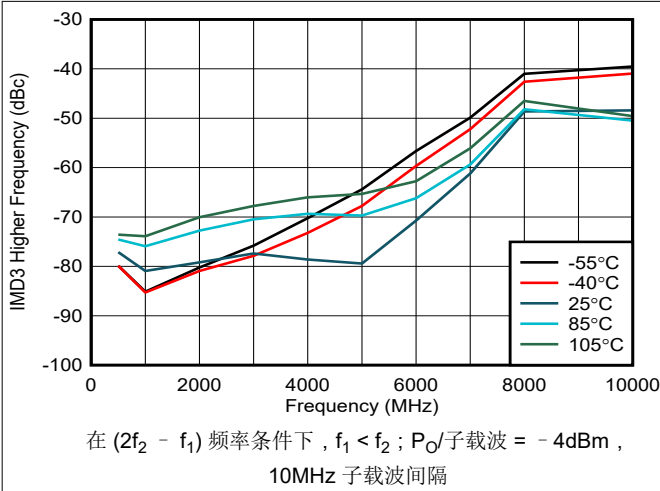
图 5-11. 整个温度范围内的 IMD3 更高
