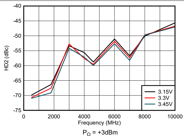
图 5-22. 整个 V_{DD} 范围内的 HD2
