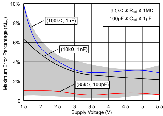
图 5-22. 电源电压范围内的最大输出脉冲宽度误差 (绝对值)
