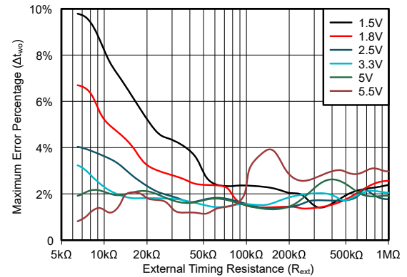
图 5-23. C_{ext} = 100\text{pF} 时最大输出脉冲宽度误差 (绝对值) 与时序电阻器值间的关系
