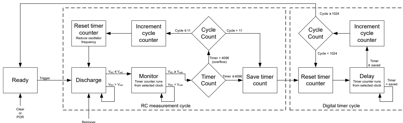
图 7-2. 状态机图
