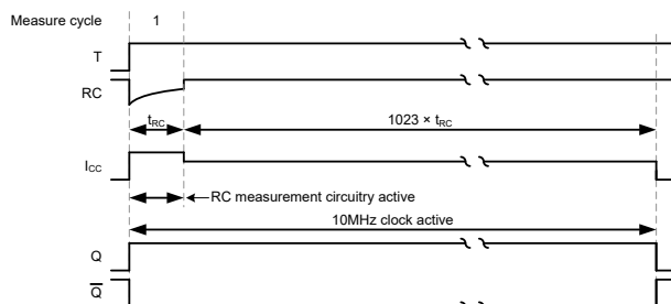
图 8-6. KRC < 400μs 的时序图
