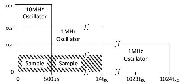
图 8-4. 较大 RC 值的活动状态功耗模式
