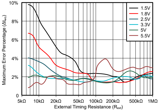
图 5-22. C_{ext} = 100pF 时最大输出脉冲宽度误差 ( 绝对值 ) 与时序电阻器值间的关系
