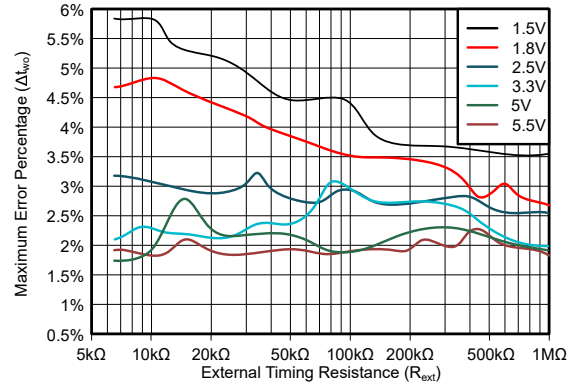
图 5-23. C_{ext} = 1nF 时最大输出脉冲宽度误差 ( 绝对值 ) 与时序电阻器值间的关系
