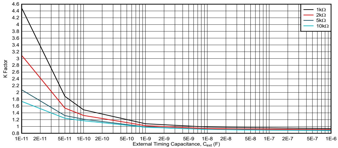
图 5-15. K 系数, V_{CC} = 5V , R_{ext} = 1k\Omega 至 10k\Omega
