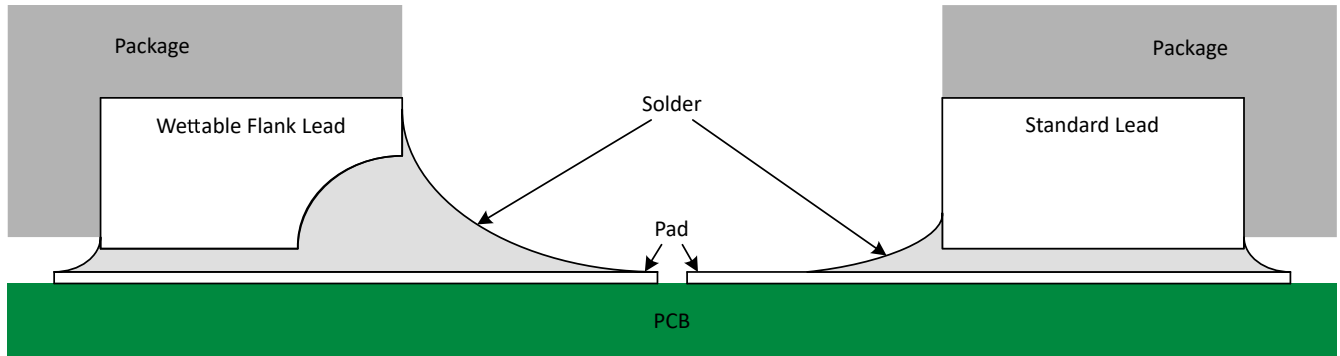
图 7-6. 焊接后具有可润湿侧翼的 QFN 封装和标准 QFN 封装的简化剖面图
