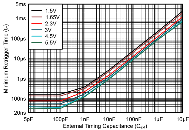
图 5-19. 最短重触发时间与外部时序电容器值间的关系
