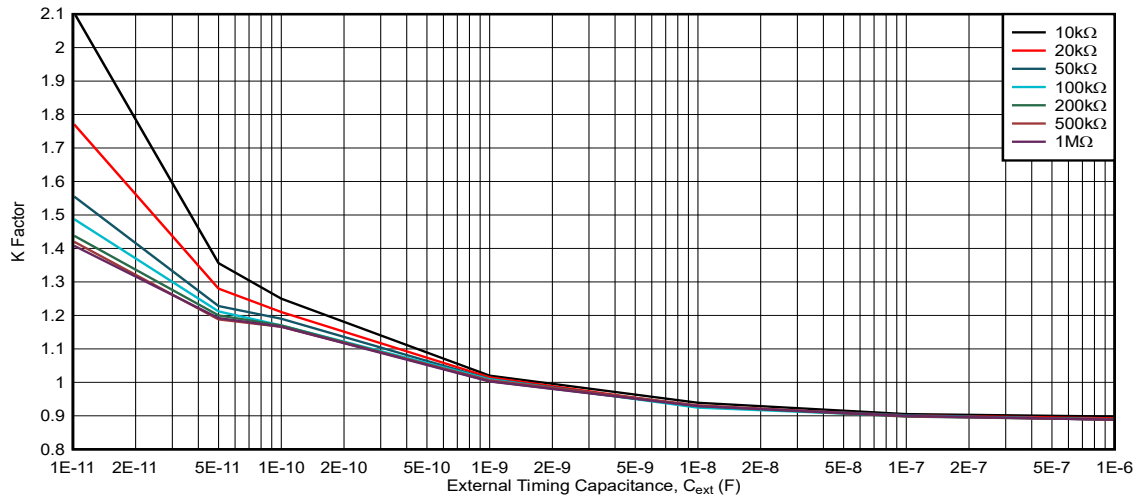
图 5-12. K 系数, V_{CC} = 2.5V , R_{ext} = 10k\Omega 至 1M\Omega
