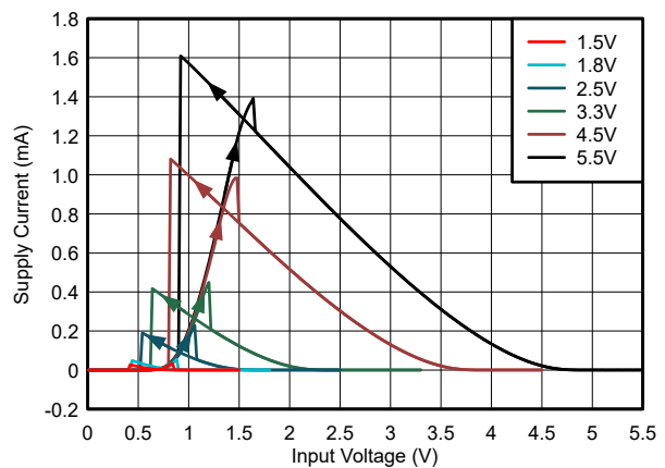
图 5-2. 电源电流与输入电压间的关系
