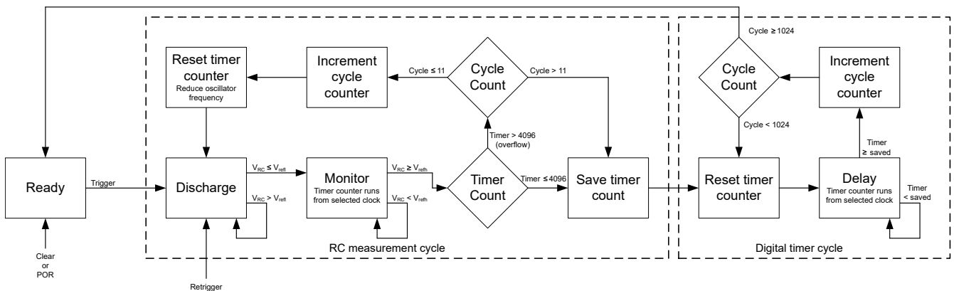
图 7-3. 状态机图
