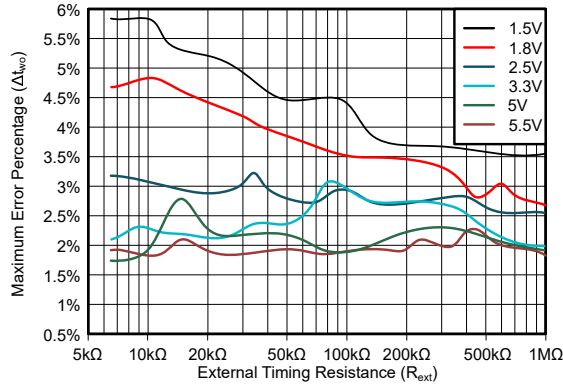
图 5-24. C_{ext} = 1nF 时最大输出脉冲宽度误差 (绝对值) 与时序电阻器值间的关系
