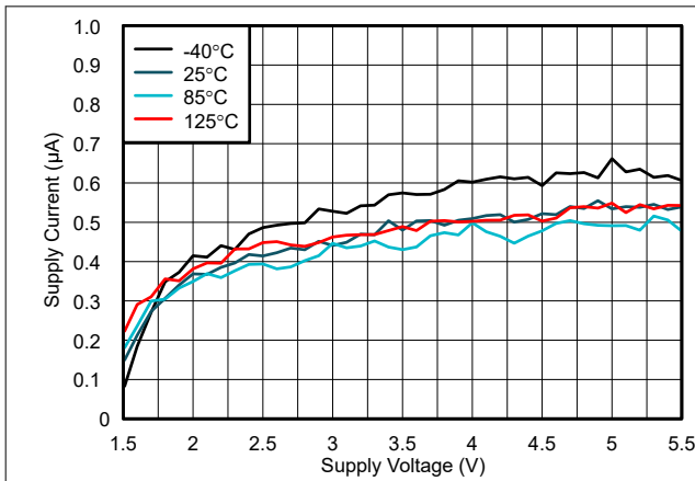
图 5-2. 电源电流与电源电压间的关系
