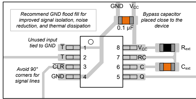
图 8-3. 布局示例
