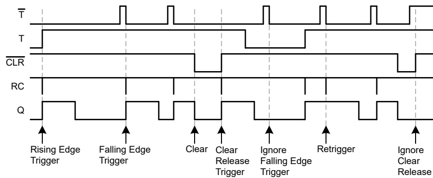
图 5-1. 时序图
