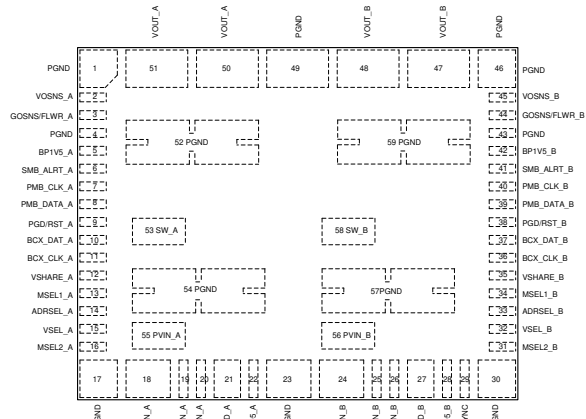
图 5-1. 59-Pin QFM-MOW Package (Top View)
