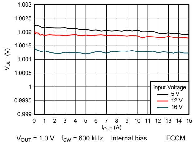
图 8-13. Load Regulation
