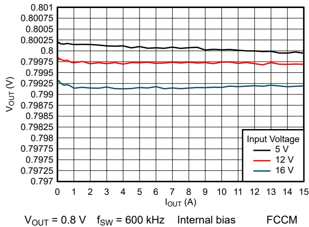
图 8-12. Load Regulation
