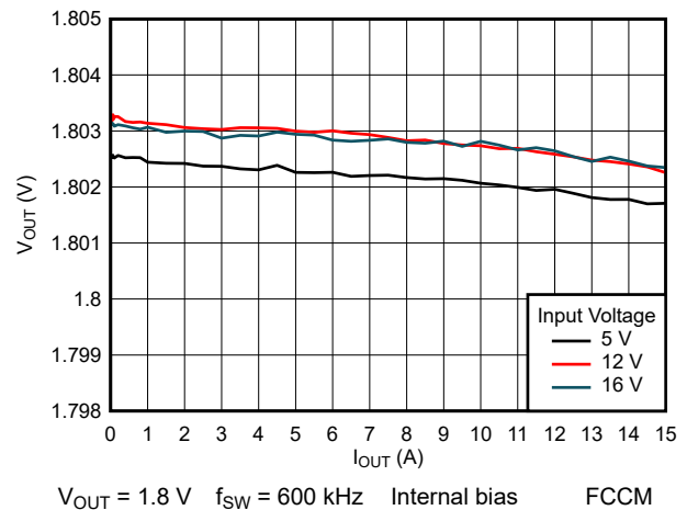
图 8-15. Load Regulation
