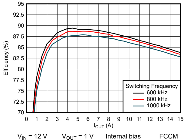
图 8-10. Efficiency
