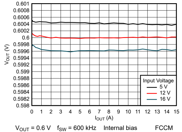
图 8-11. Load Regulation
