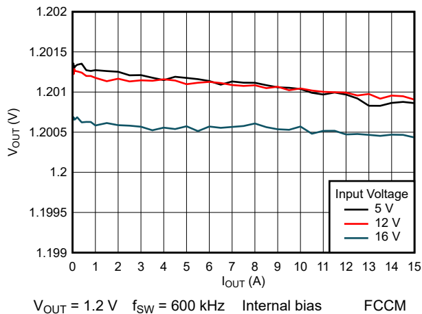
图 8-14. Load Regulation
