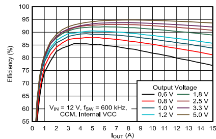
效率图
