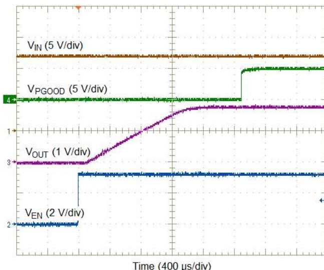
图 13. Enable Turnon
