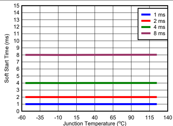
图 6-12. 软启动
