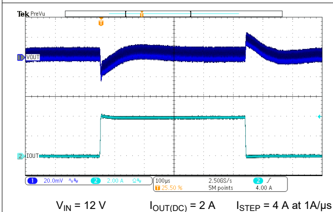
图 7-8. Load Transient
