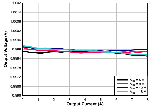
图 7-5. Load Regulation
