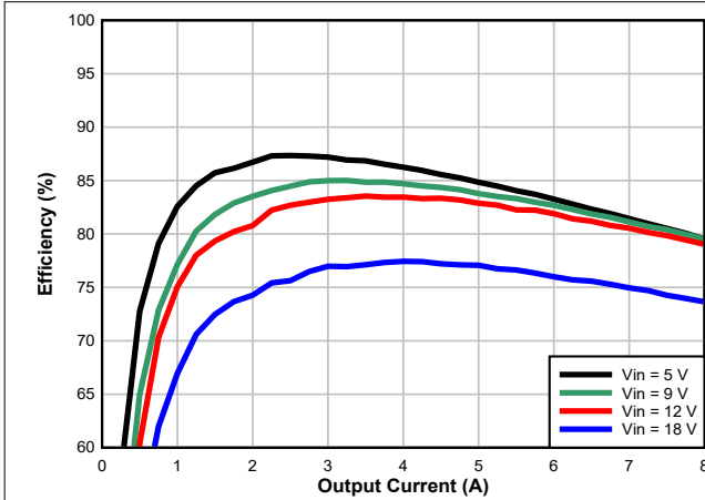
图 7-4. Efficiency
