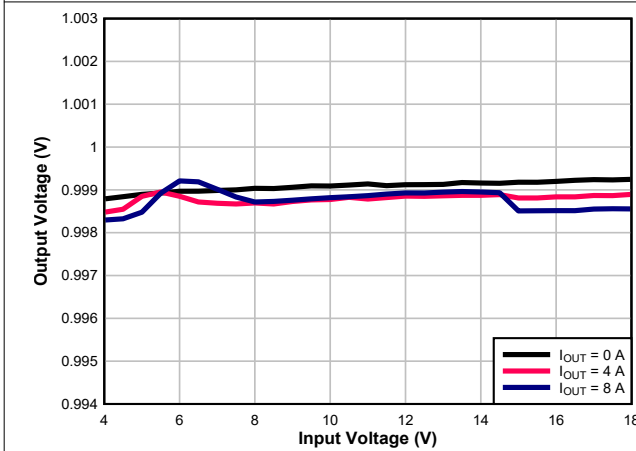
图 7-6. Line Regulation
