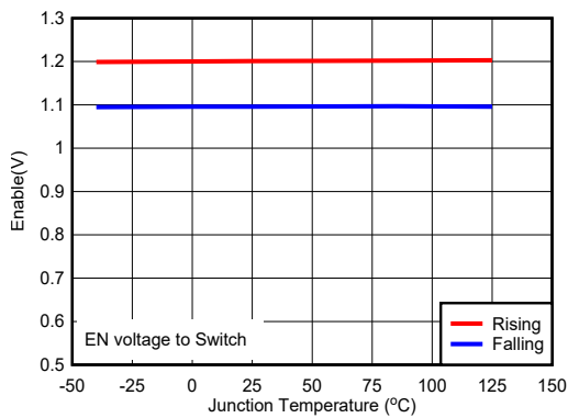
图 5-5. Enable Voltage
