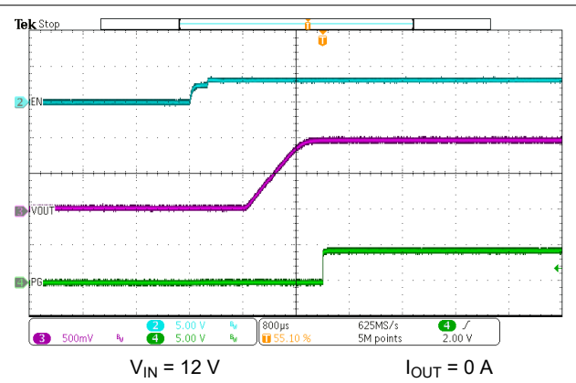
图 7-9. EN Start-Up - No Load
