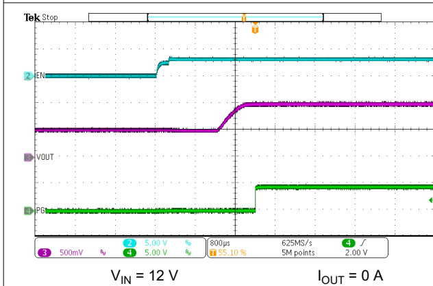
图 7-12. EN Start-Up - 0.5-V Prebias
