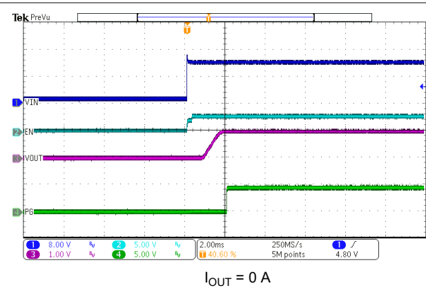
图 7-13. VIN Start-Up
