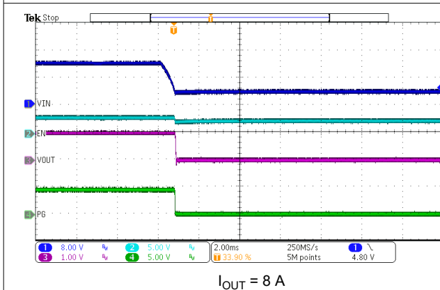
图 7-14. VIN Shutdown
