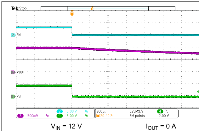
图 7-10. EN Shutdown No Load
