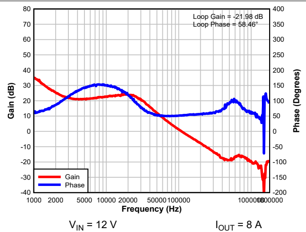
图 7-7. Bode Plot
