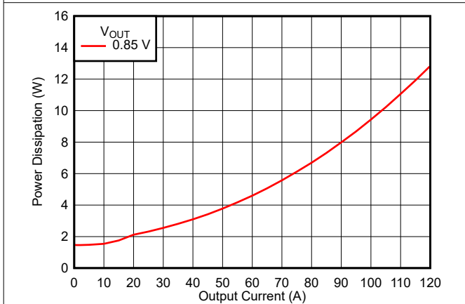
图 8-4. VOUTA Power Dissipation
