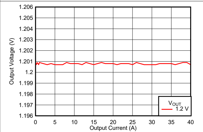
图 8-7. VOUTB Load Regulation
