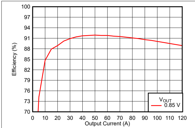
图 8-2. VOUTA Efficiency
