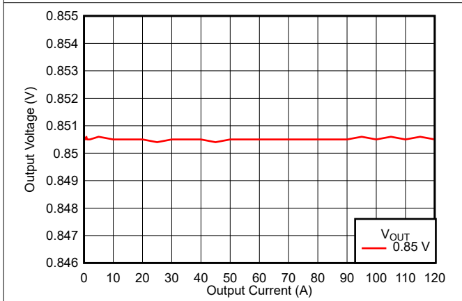
图 8-6. VOUTA Load Regulation
