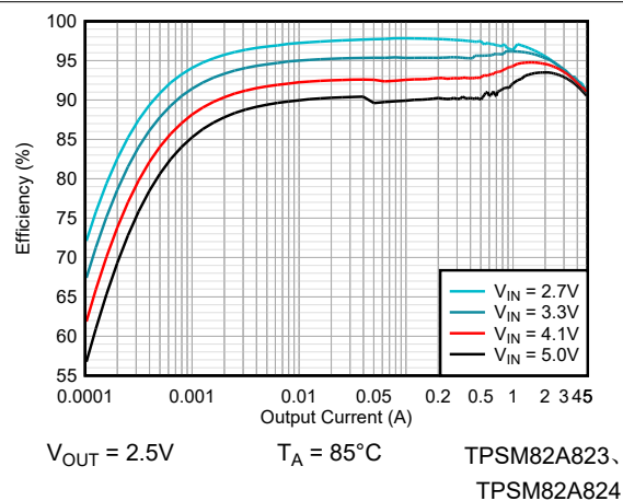
图 8-5. 效率
