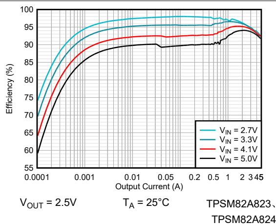
图 8-4. 效率
