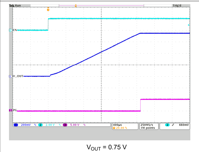
图 9-35. Start-Up Using EN Pin
