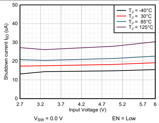
图 6-2. Shutdown Current
