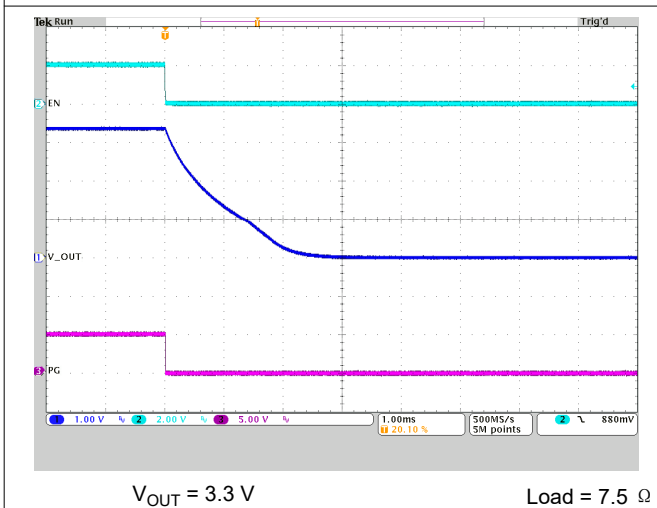
图 9-36. Shutdown Using EN Pin (Discharge Enabled)
