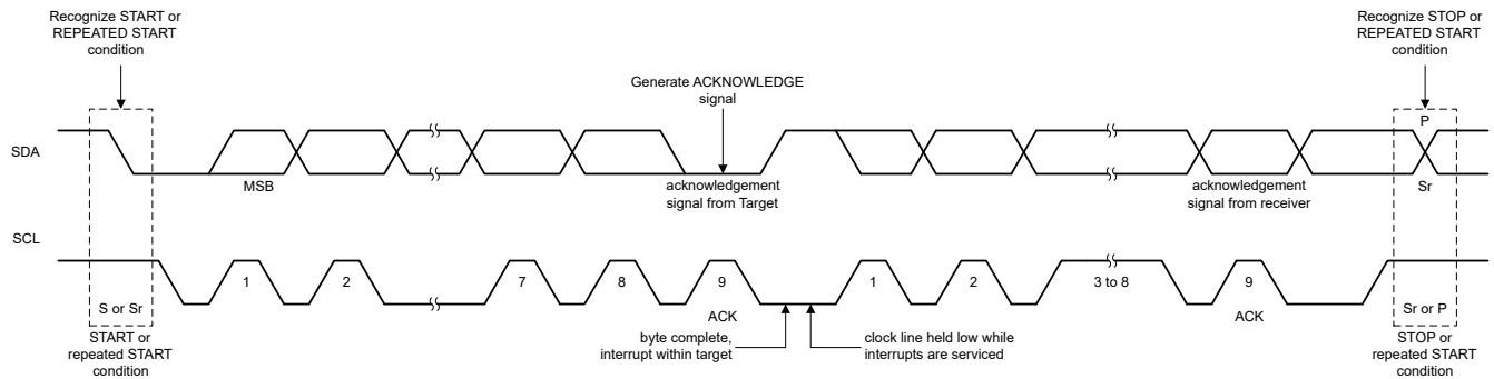
图 7-26. Bus Protocol
