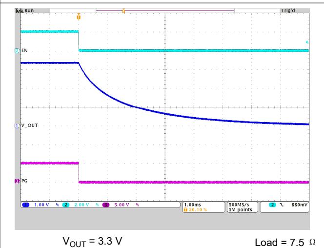
图 9-37. Shutdown Using EN Pin (Discharge Disabled)
