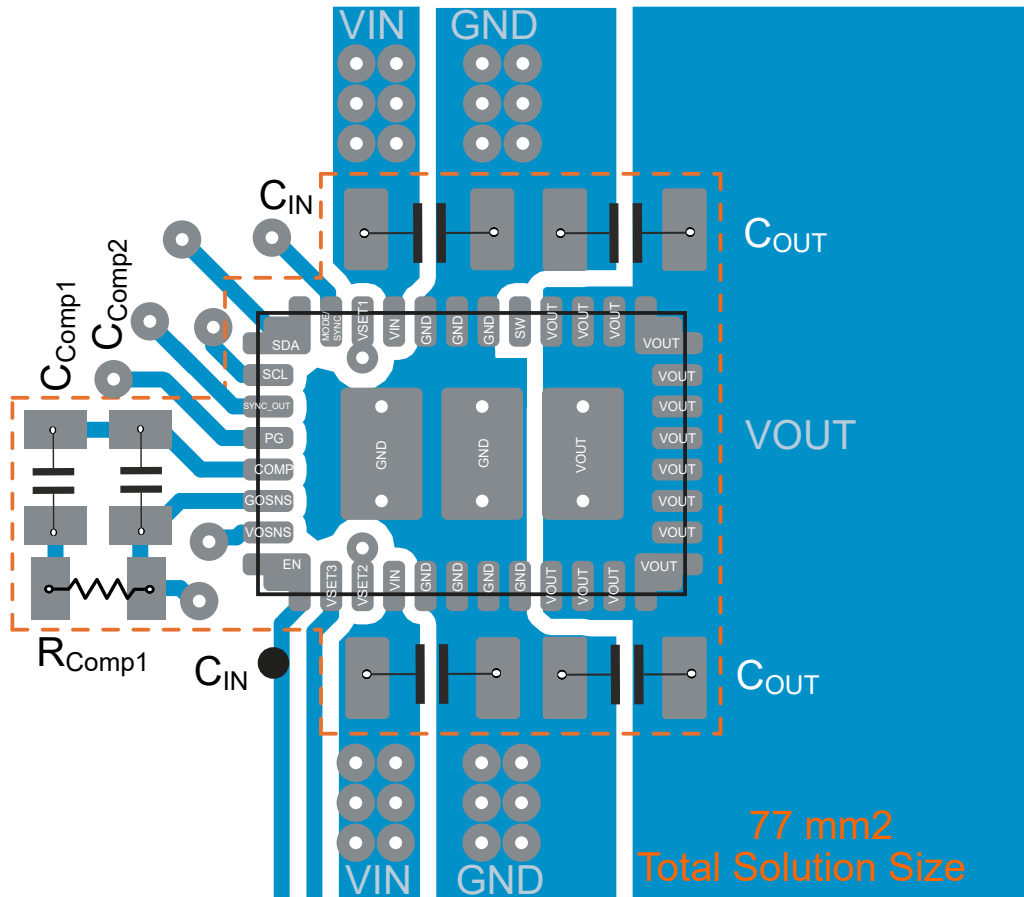
图 9-57. Layout Example
