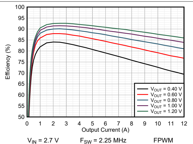
图 9-9. Efficiency TPSM8287A12BBS
