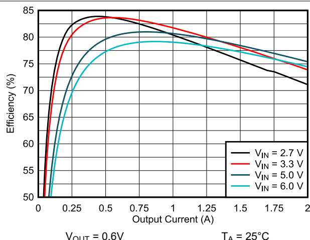
图 9-11. 效率与输出电流间的关系
