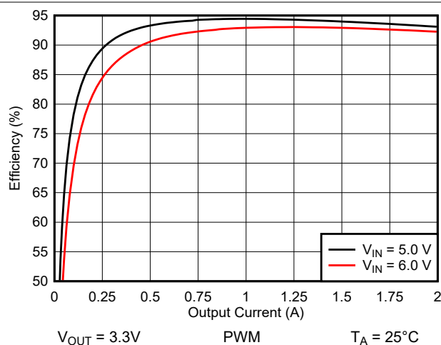
图 9-3. 效率与输出电流间的关系
