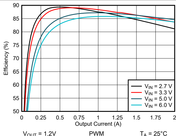
图 9-9. 效率与输出电流间的关系
