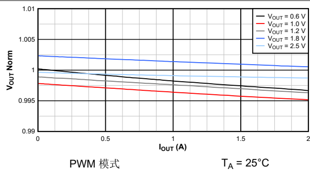
图 9-13. 负载调整率 ( V_{IN} = 3.3\text{ V} )
