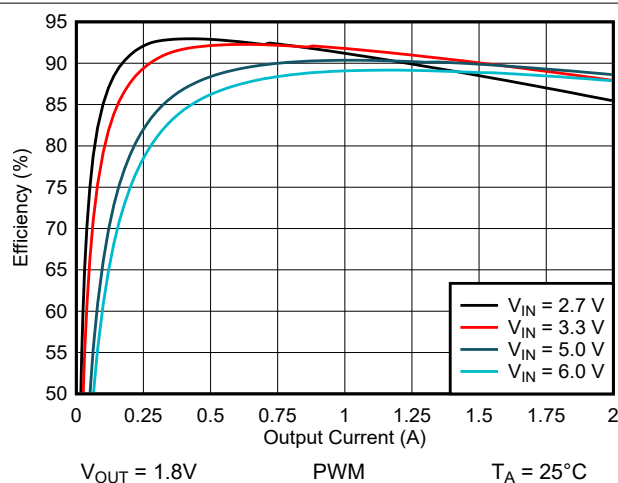
图 9-7. 效率与输出电流间的关系
