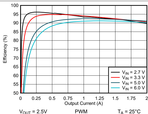
图 9-5. 效率与输出电流间的关系
