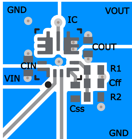
图 9-33. 布局示例
