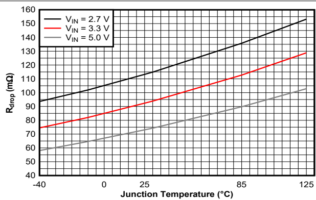
图 6-1. 压降电阻
