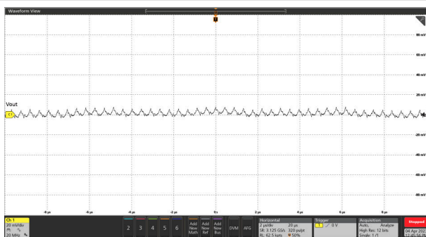
图 9-20. 输出和输入电压纹波
