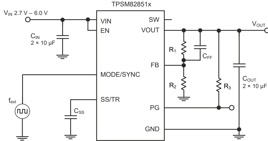
图 9-30. 频率同步
