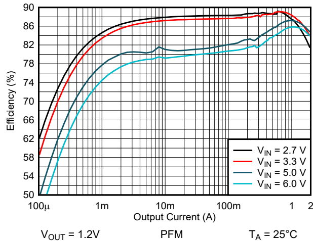
图 9-8. 效率与输出电流间的关系
