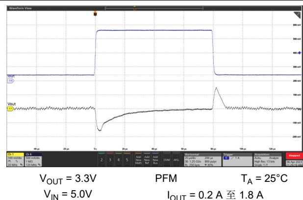
图 9-19. 负载瞬态响应
