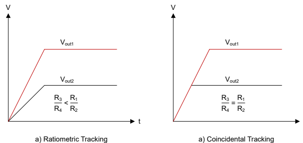
图 9-29. 输出电压跟踪
