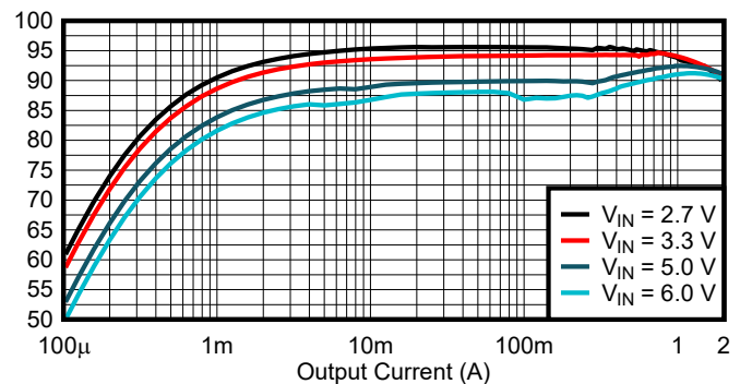
效率与输出电流间的关系； V_{OUT} = 2.5V
