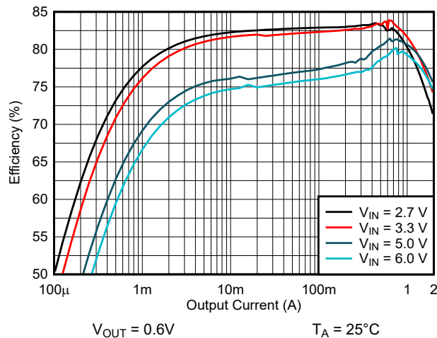
图 9-10. 效率与输出电流间的关系
