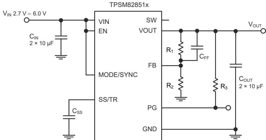
图 9-1. 典型应用原理图
