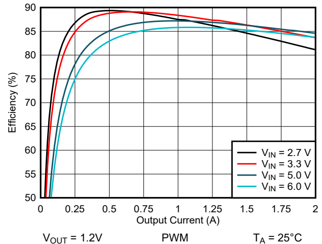
图 9-9. 效率与输出电流间的关系
