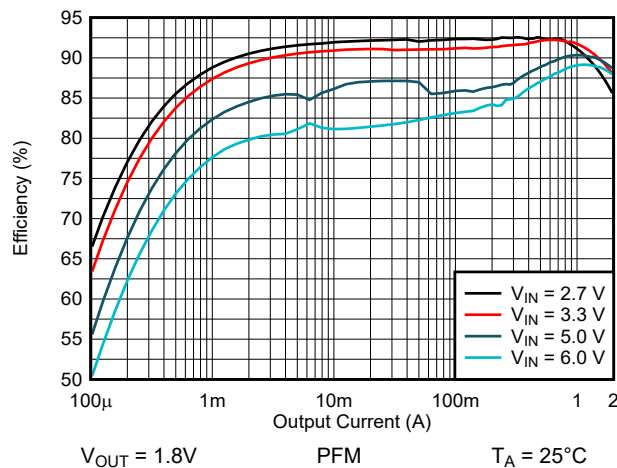
图 9-6. 效率与输出电流间的关系
