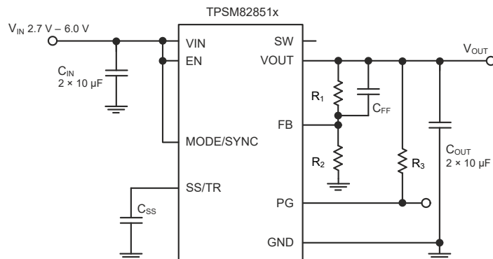
图 7-1. TPSM82851x 的测量设置
