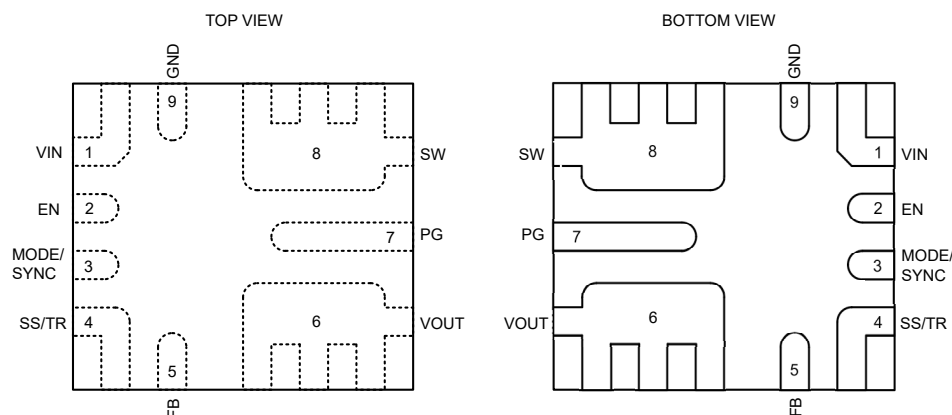
图 5-1.9 引脚 RDY QFN 封装
