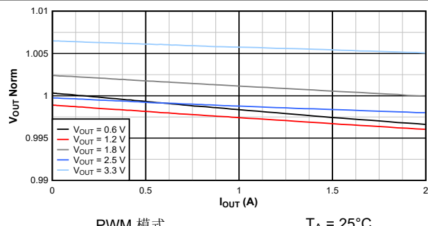
图 9-15. 负载调整率 ( V_{IN} = 5V )
