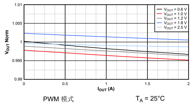
图 9-13. 负载调整率 ( V_{IN} = 3.3\text{ V} )
