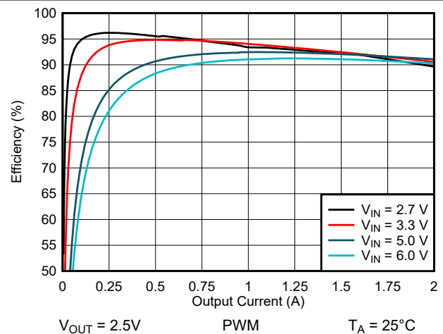
图 9-5. 效率与输出电流间的关系
