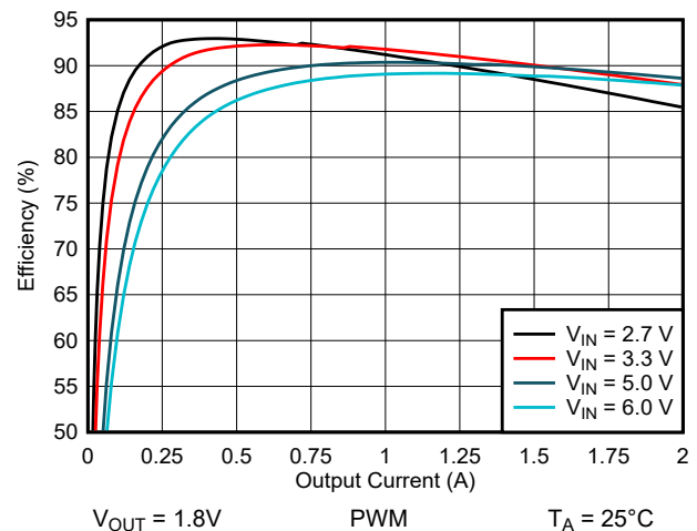
图 9-7. 效率与输出电流间的关系
