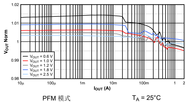
图 9-12. 负载调整率 ( V_{IN} = 3.3\text{ V} )
