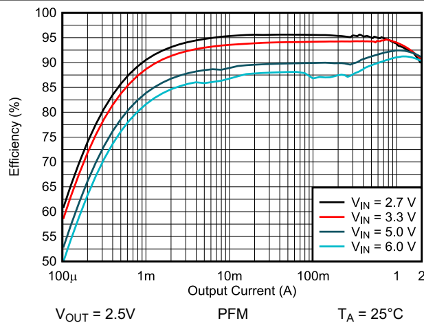
图 9-4. 效率与输出电流间的关系
