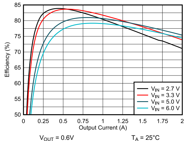
图 9-11. 效率与输出电流间的关系
