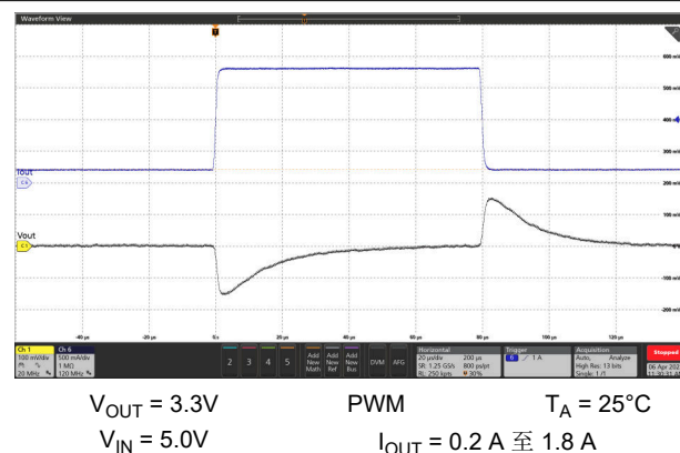
图 9-18. 负载瞬态响应
