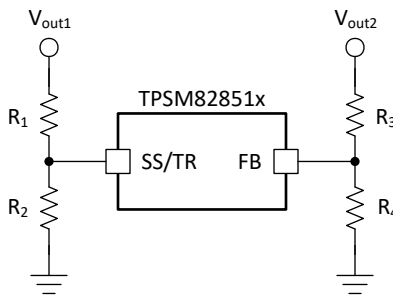
图 9-28. 输出电压跟踪原理图
