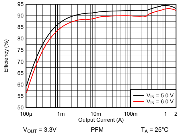
图 9-2. 效率与输出电流间的关系
