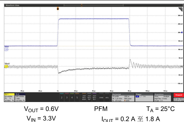
图 9-17. 负载瞬态响应
