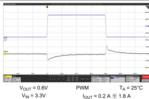
图 9-16. 负载瞬态响应
