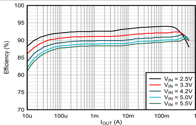
图 8-8. 效率 (1.8V V_{OUT} 和 25°C)
