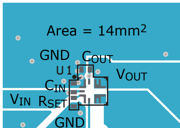
图 8-34. 布局示例
