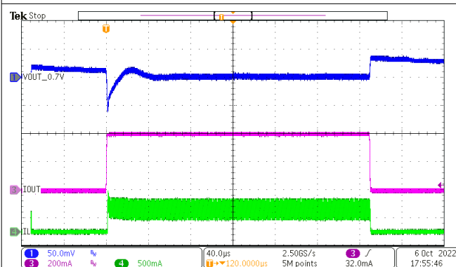
图 8-22. 负载瞬态 ( 0.7V V_{OUT} 、 I_{OUT} = 100\mu A 至 400mA )
