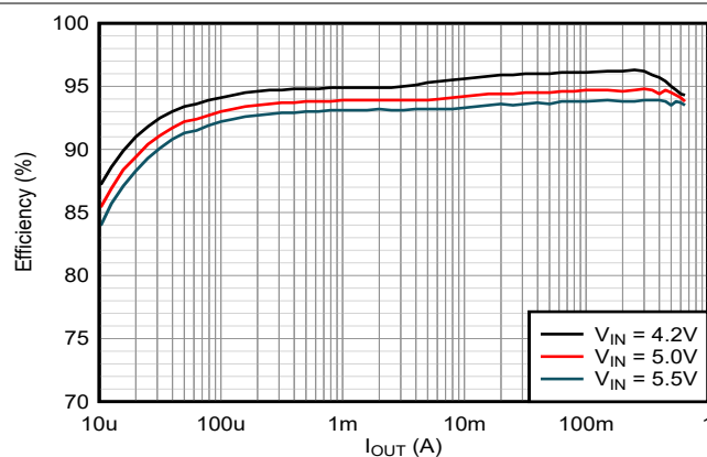
图 8-11. 效率 (3.6V V_{OUT} 和 85°C)
