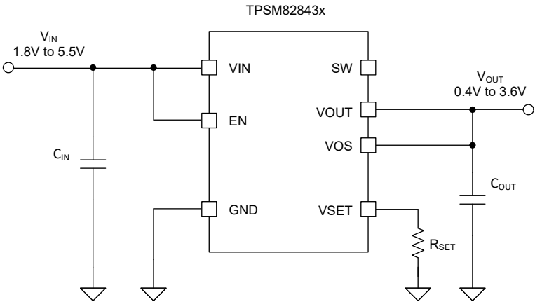
图 8-1. TPSM82843 典型应用电路
