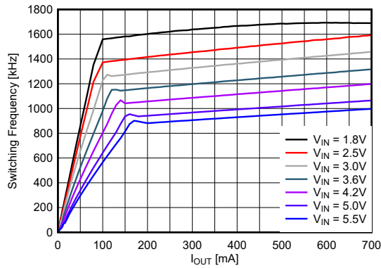
图 8-14. 开关频率与输出电流间的关系 (0.4V V_{OUT} )
