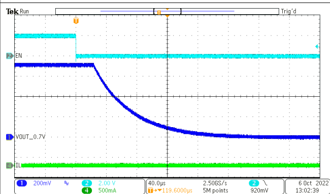
图 8-31. 关断、输出放电 ( 0.7V V_{OUT} )
