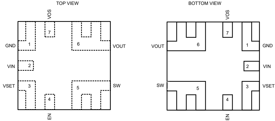
图 5-1. VCF, 7 引脚 QFN-FCMOD 封装
