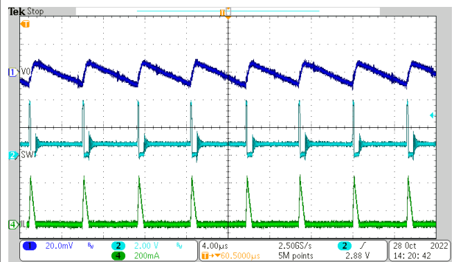
图 8-19. 典型运行情况 (0.7V V_{OUT} 、20mA I_{OUT} )
