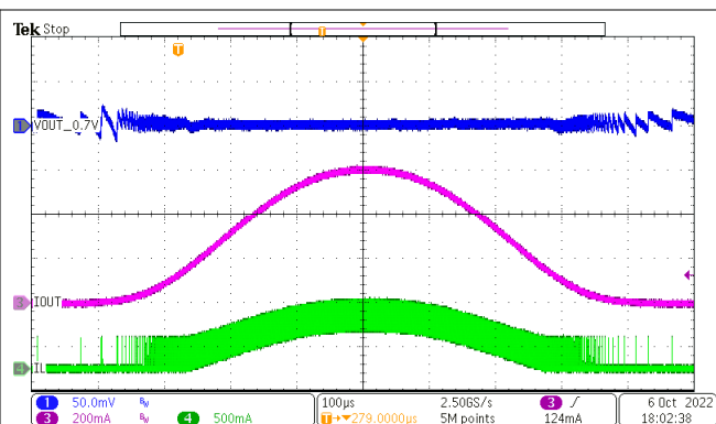
图 8-27. 交流负载扫描 ( 0.7V V_{OUT} 、 I_{OUT} = 1mA 至 600mA )
