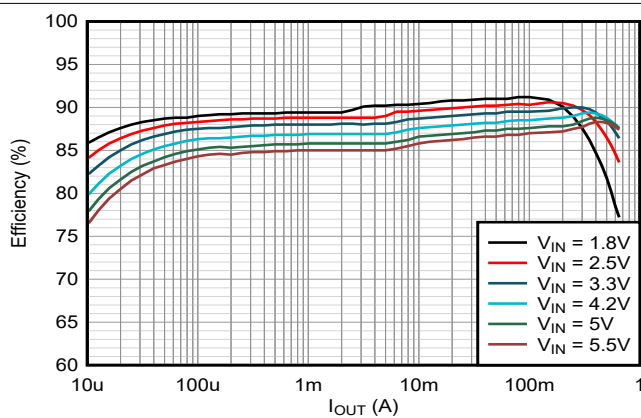
图 8-6. 效率 (1.2V V_{OUT} 和 25°C)
