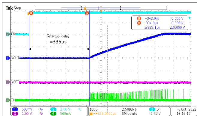
图 8-32. 启动延迟时间 ( VSET = GND )
