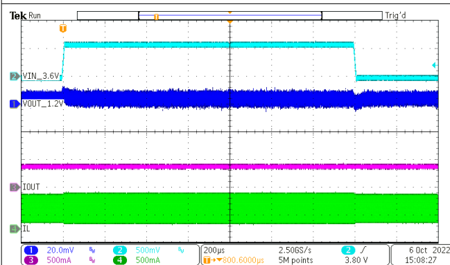
图 8-30. 线路瞬态 ( 1.2V V_{OUT} 、 I_{OUT} = 400mA、 V_{IN} = 3.6V 至 4.2V )
