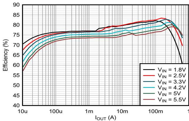
图 8-2. 效率 (0.4V V_{OUT} 和 25°C)
