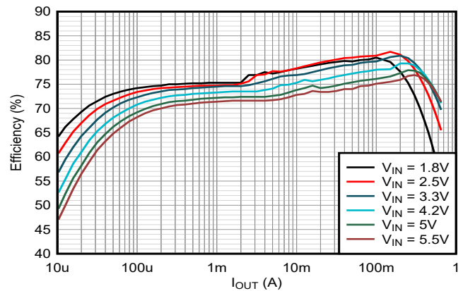
图 8-3. 效率 (0.4V V_{OUT} 和 85°C)
