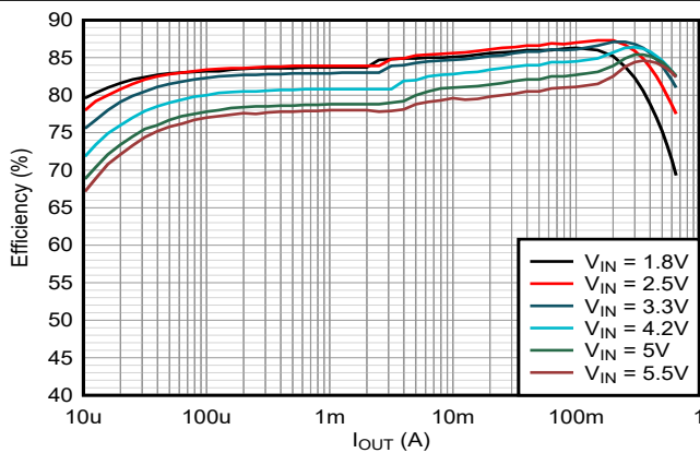
图 8-4. 效率 (0.7V V_{OUT} 和 25°C)
