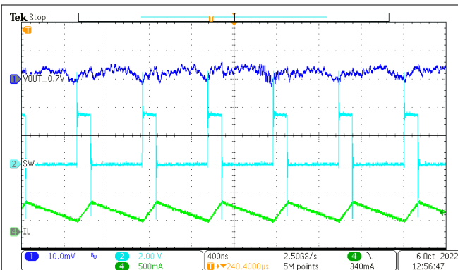
图 8-20. 典型运行情况 ( 0.7V V_{OUT} 、400mA I_{OUT} )
