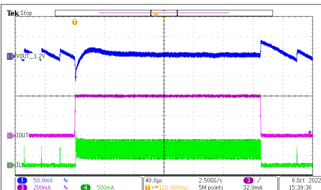
图 8-26. 负载瞬态 ( 1.2V V_{OUT} 、 I_{OUT} = 5mA 至 400mA )
