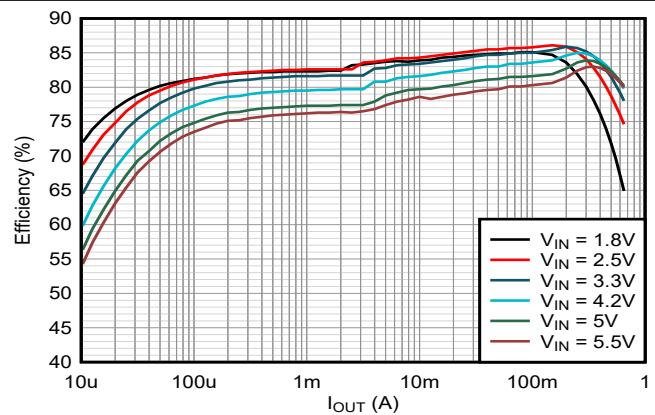
图 8-5. 效率 (0.7V V_{OUT} 和 85°C)
