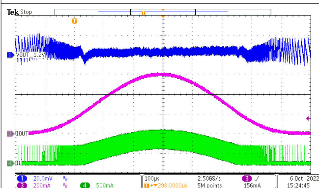
图 8-28. 交流负载扫描 ( 1.2V V_{OUT} 、 I_{OUT} = 1mA 至 600mA )
