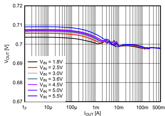
图 8-13. 输出电压与输出电流间的关系 (0.7V V_{OUT} )
