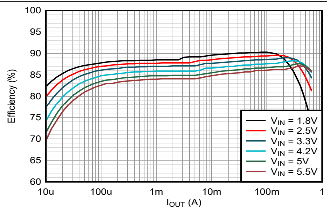
图 8-7. 效率 (1.2V V_{OUT} 和 85°C)
