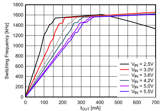
图 8-17. 开关频率与输出电流间的关系 (1.8V V_{OUT} )
