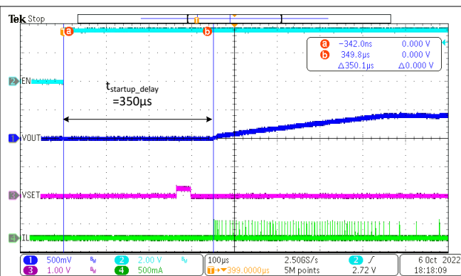
图 8-33. 启动延迟时间 ( VSET = 10kΩ )
