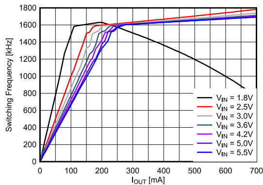
图 8-16. 开关频率与输出电流间的关系 (1.2V V_{OUT} )
