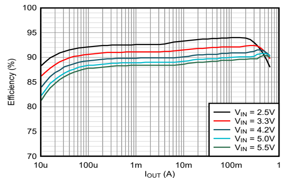
效率与输出电流间的关系曲线 (电压为 1.8V_{OUT} 时)
