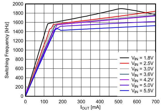
图 8-15. 开关频率与输出电流间的关系 (0.7V V_{OUT} )
