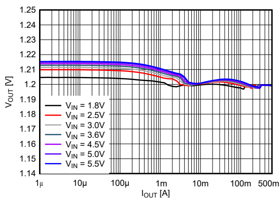
图 8-12. 输出电压与输出电流间的关系 (1.2V V_{OUT} )
