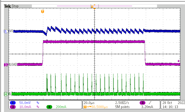
图 8-24. 负载瞬态 ( 1.2V V_{OUT} 、 I_{OUT} = 100\mu A 至 20mA )
