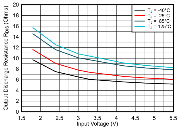
图 6-4. VOS 放电开关漏源电阻 R_{DIS}
