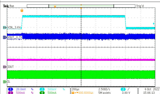
图 8-29. 线路瞬态 ( 0.7V V_{OUT} 、 I_{OUT} = 400mA、 V_{IN} = 3.6V 至 4.2V )
