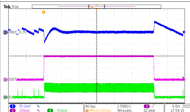
图 8-23. 负载瞬态 ( 0.7V V_{OUT} 、 I_{OUT} = 5mA 至 400mA )
