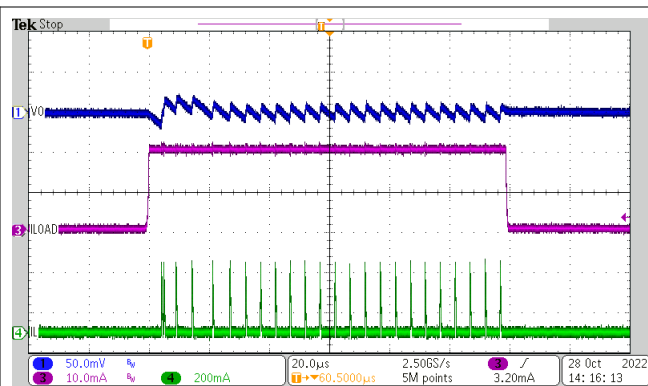
图 8-21. 负载瞬态 ( 0.7V V_{OUT} 、 I_{OUT} = 100\mu A 至 20mA )
