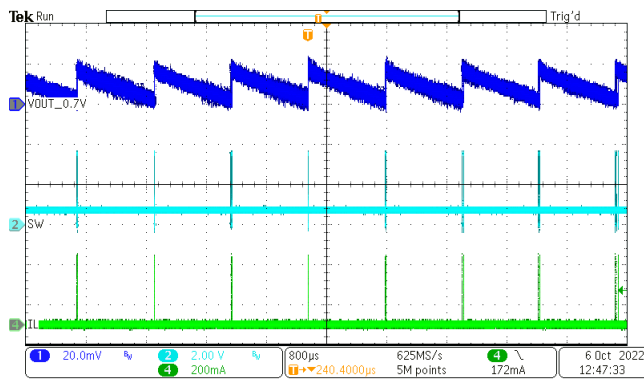
图 8-18. 典型运行情况 (0.7V V_{OUT} 、100 \mu A I_{OUT} )
