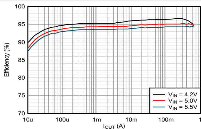
图 8-10. 效率 (3.6V V_{OUT} 和 25°C)
