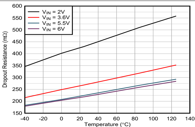
图 6-3. 压降电阻 R_{DS(ON)}
