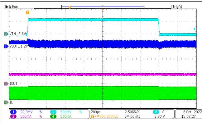
图 8-25. 负载瞬态 ( 1.2V V_{OUT} 、 I_{OUT} = 100\mu A 至 400mA )
