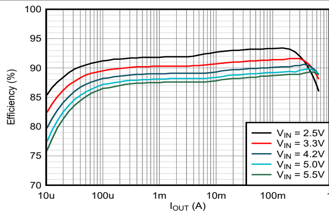
图 8-9. 效率 (1.8V V_{OUT} 和 85°C)
