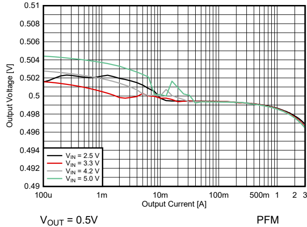
图 8-14. 输出电压与输出电流间的关系
