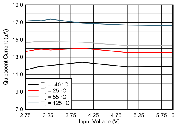
图 6-1. Quiescent Current
