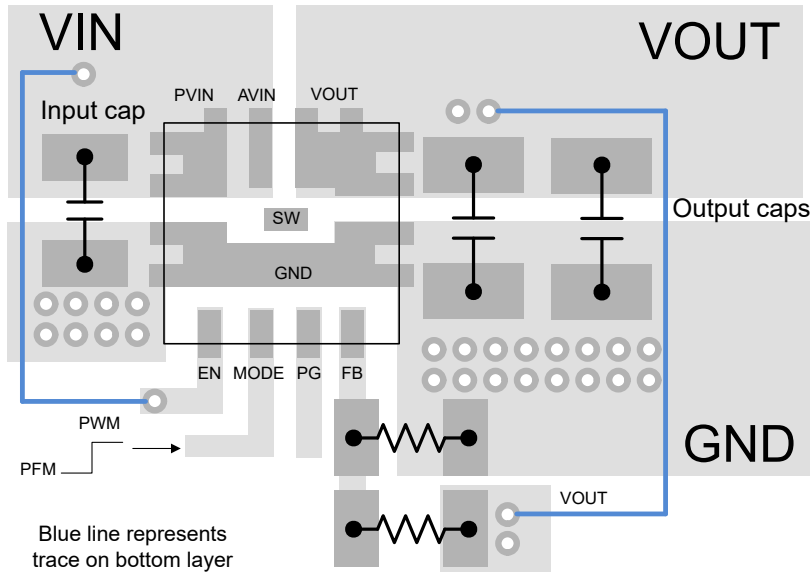
图 7-15. 布局示例
