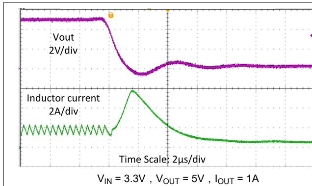
图 7-11. 输出短路保护 (进入)
