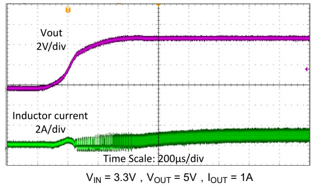
图 7-12. 输出短路保护 (恢复)
