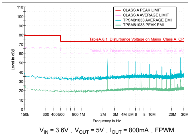
图 7-13. 传导 EMI 性能 (CISPR32)
