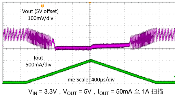
图 7-9. 负载扫描
