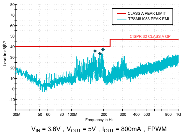
图 7-14. 辐射 EMI 性能 (CISPR32)
