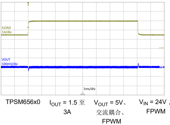
图 8-15. 负载瞬态 ( 50 至 100% )
