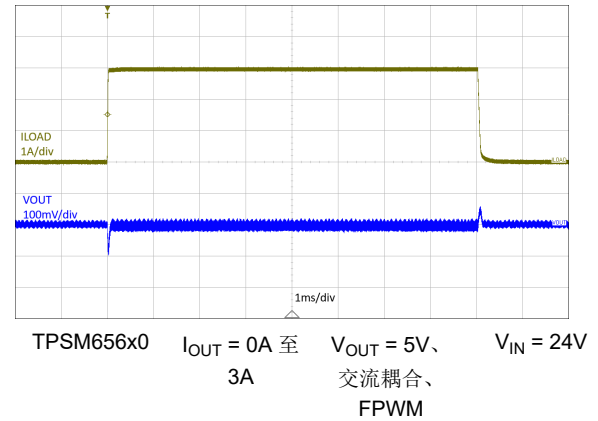
图 8-14. 负载瞬态 ( 0 至 100% )
