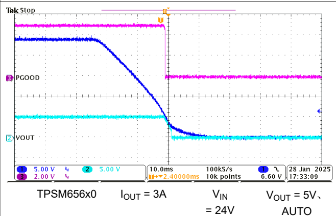
图 8-10. 关断
