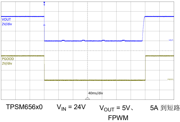
图 8-13. 应用短路
