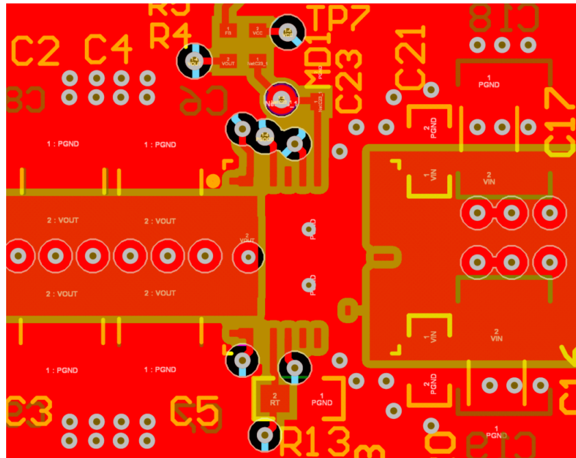
图 8-20. 布局示例
