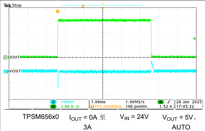
图 8-8. 负载瞬态 (0% 至 100%)
