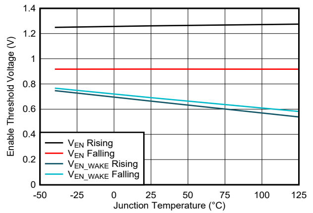
图 6-6. 使能阈值
