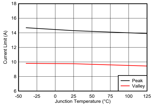
图 6-4. 高侧 (峰值) 和低侧 (谷值) 电流限制 TPSM63610
