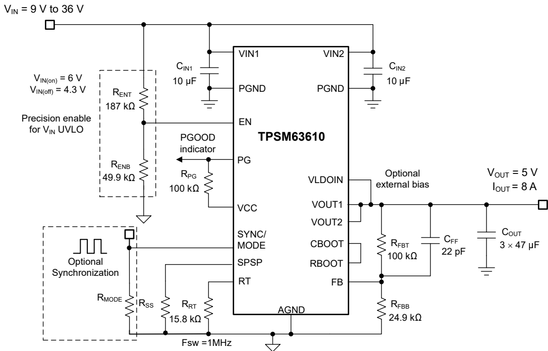
图 8-1. 电路原理图
