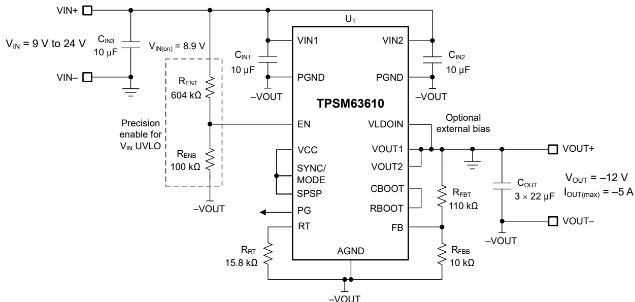
图 8-14. 电路原理图
