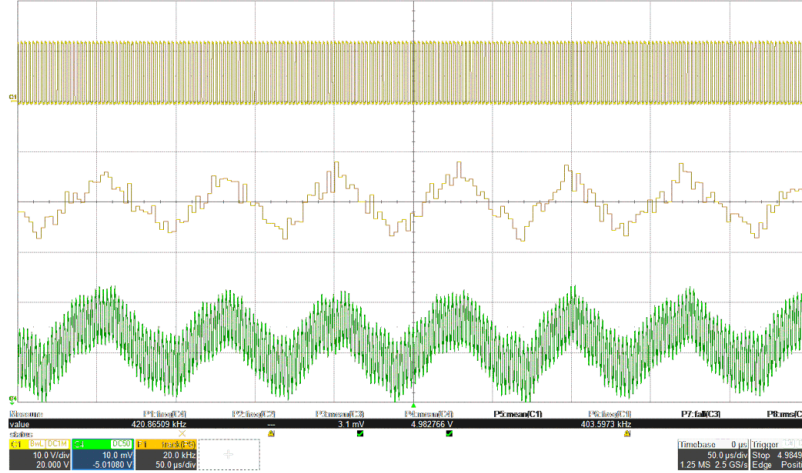
图 7-3. 没有纹波消除功能的输出纹波显示 V_{\text{sw}} (顶部)、 F_{\text{sw}} (中间)、 V_{\text{out}} (底部)
