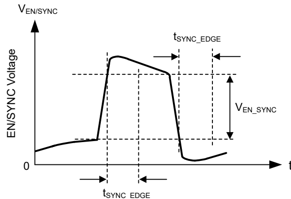
图 7-2. 典型 SYNC 波形
