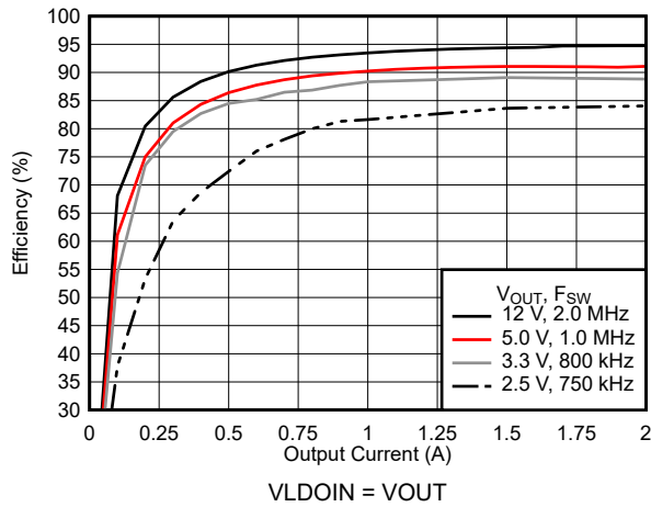
图 7-11. 效率
