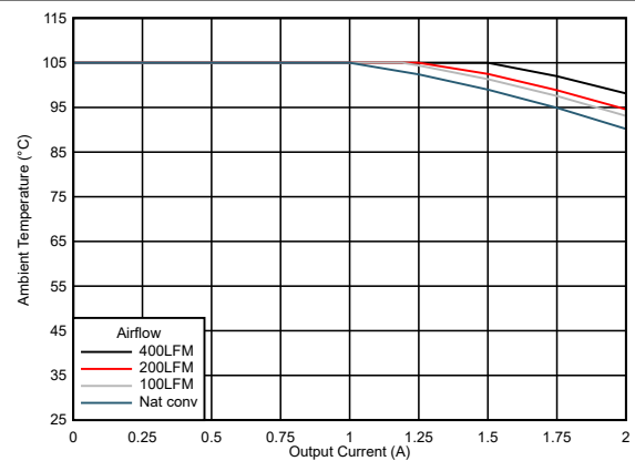
图 7-16. 安全工作区 ( V_{OUT} = 12V )
