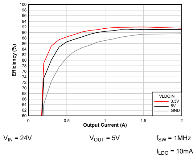
图 8-8. 通过 VLDOIN 实现的效率提升 (V OUT = 5V)
