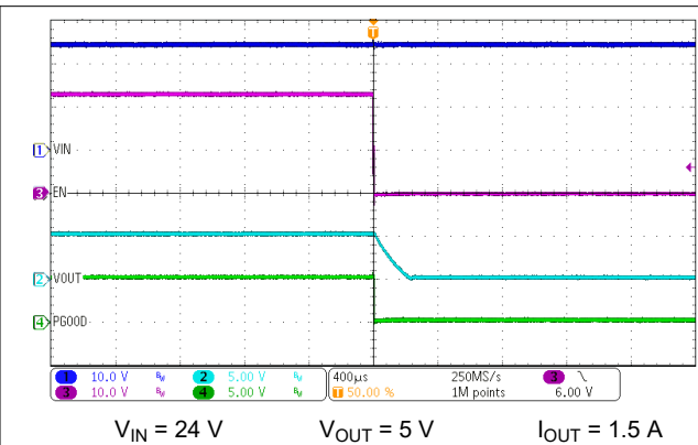
图 9-3. Enable Shutdown Waveforms
