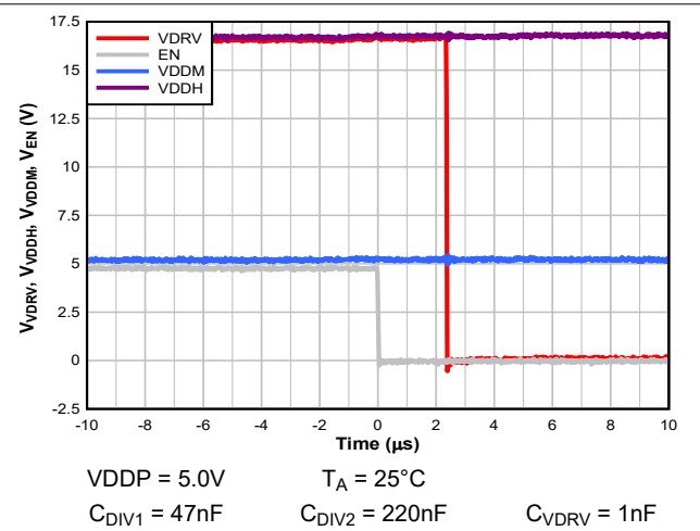
图 6-4. t_{HL\_VDRV}
