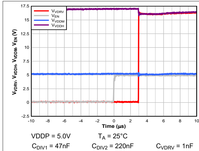
图 6-3. t_{LH\_VDRV}
