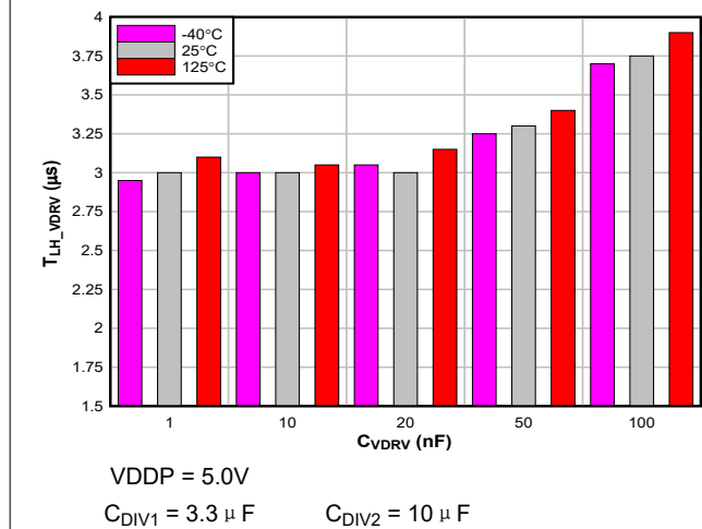
图 6-5. t_{LH\_VDRV} 与 C_{VDRV}
