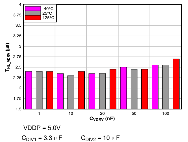
图 6-6. t_{HL\_VDRV} 与 C_{VDRV}
