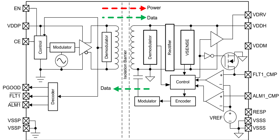
图 8-4. TPSI3133
