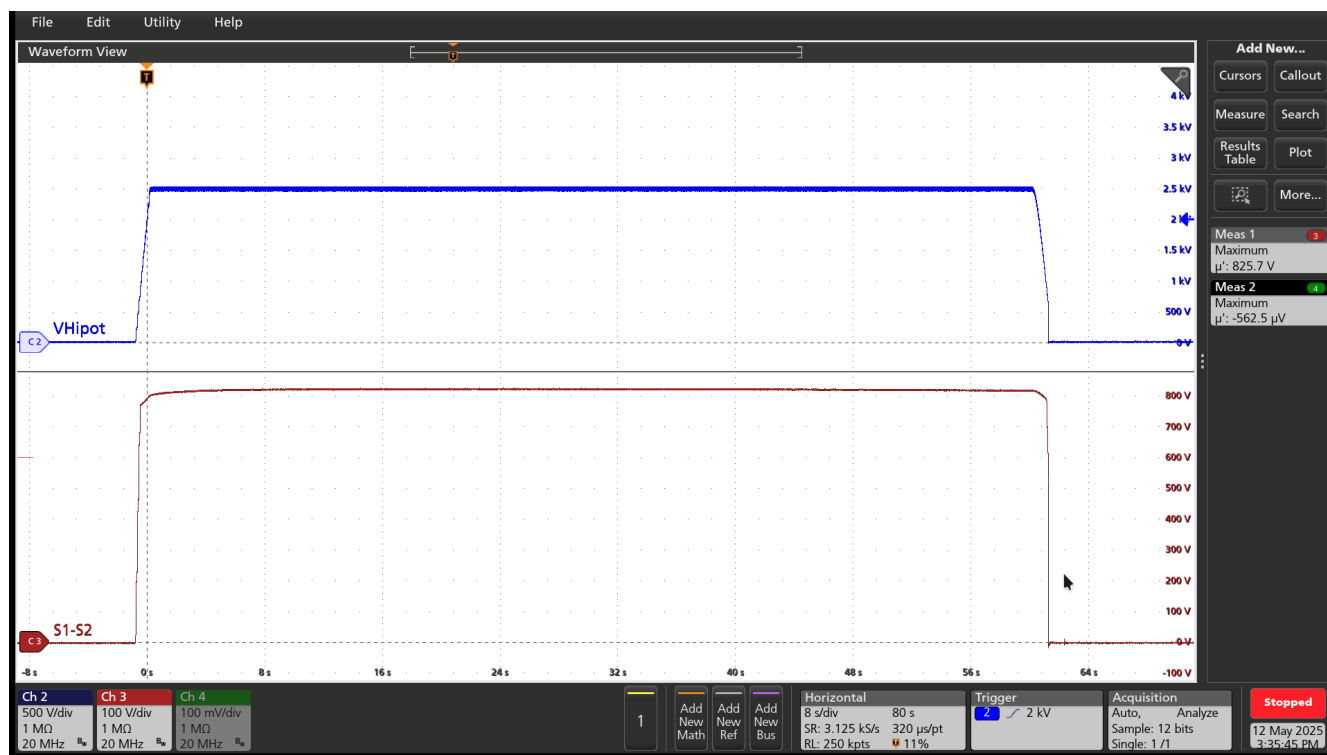
图 9-9. 在 V_{\text{HIPOT}} = 2500\text{V} 且使用 900\text{k}\Omega 限流电阻器时的雪崩电压 ( V_{\text{S1S2}} )
