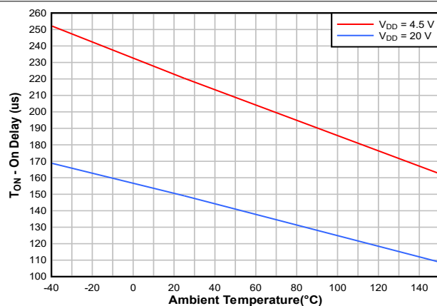
图 6-7. 输入到输出开启延迟 ( V_{IN} = 500V )
