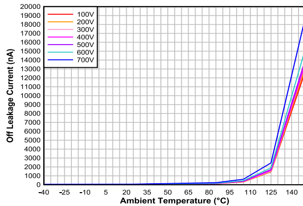
图 6-3. 关断泄漏电流与环境温度间的关系
