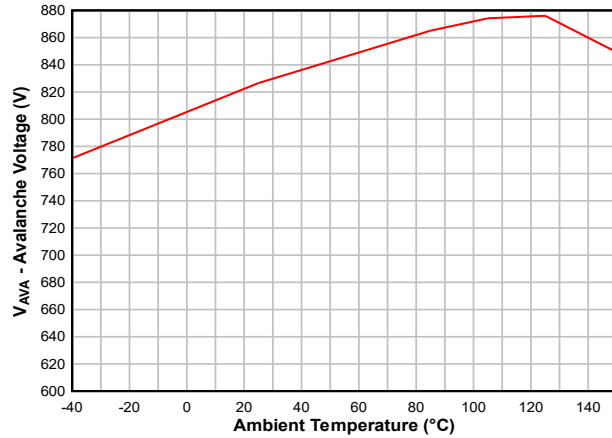
图 6-1. 雪崩电压与环境温度间的关系 ( I_O = 100uA )
