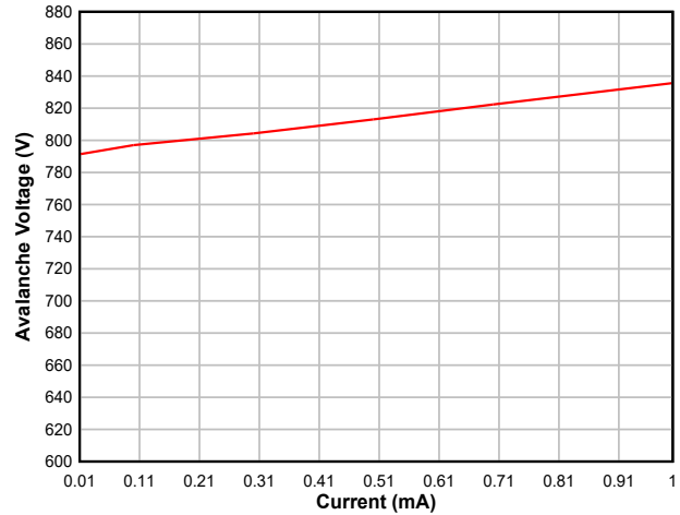
图 6-2. 雪崩电压与雪崩电流间的关系
