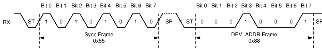
图 6-13. Synchronization Byte
