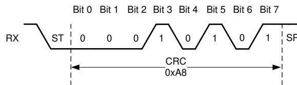
图 6-15. CRC Byte
