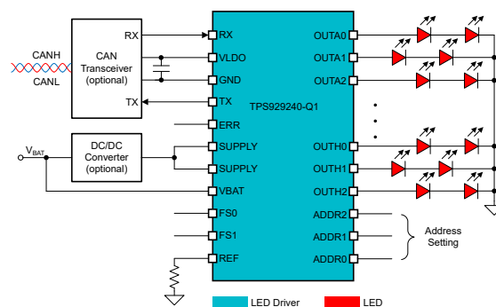
典型应用图
