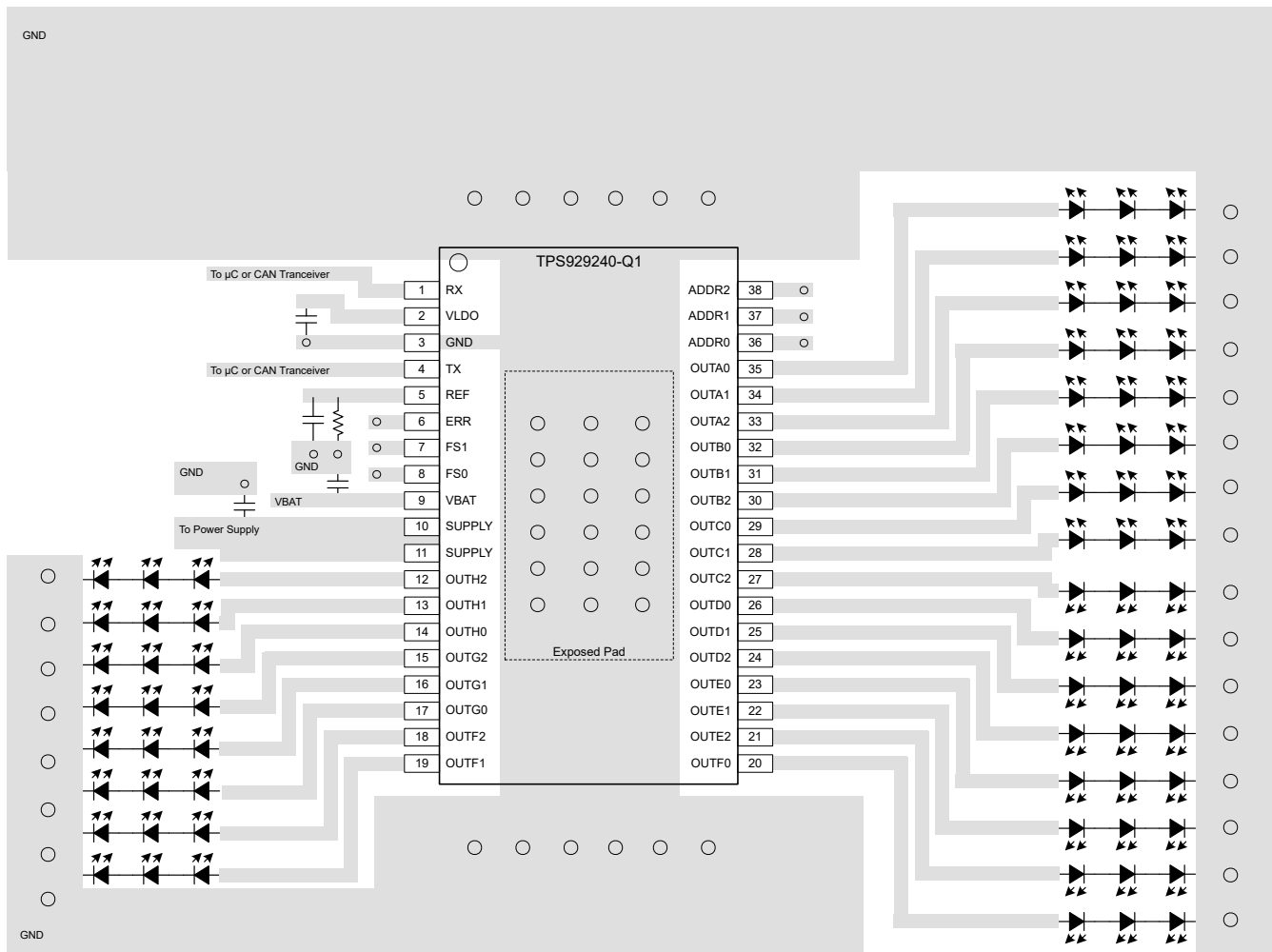
图 7-5. TPS929240-Q1 Layout
