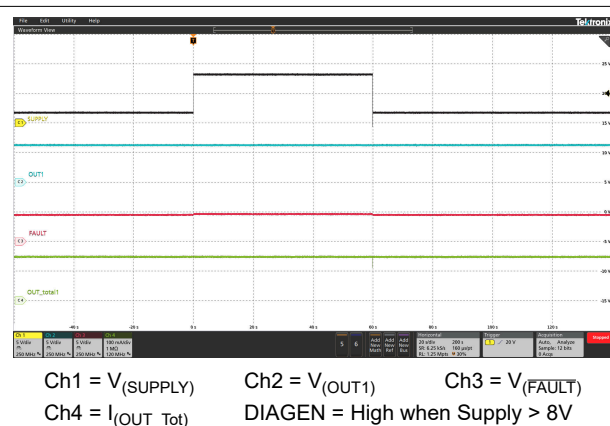
图 5-24. Jump Start
