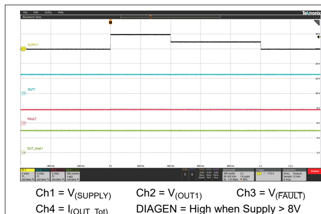
图 5-19. Transient Overvoltage
