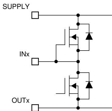
图 6-14. INx Pins
