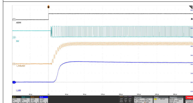
黑色： \text{DIM}_{\text{Analog}} ，浅蓝色：SW，橙色：电感器电流，深蓝色：LED 电流
