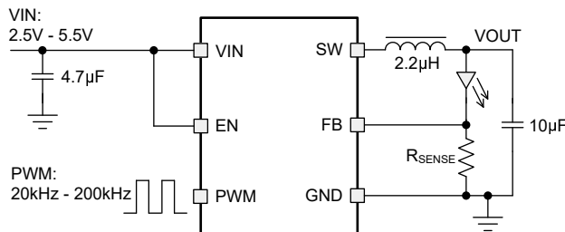
简化原理图
