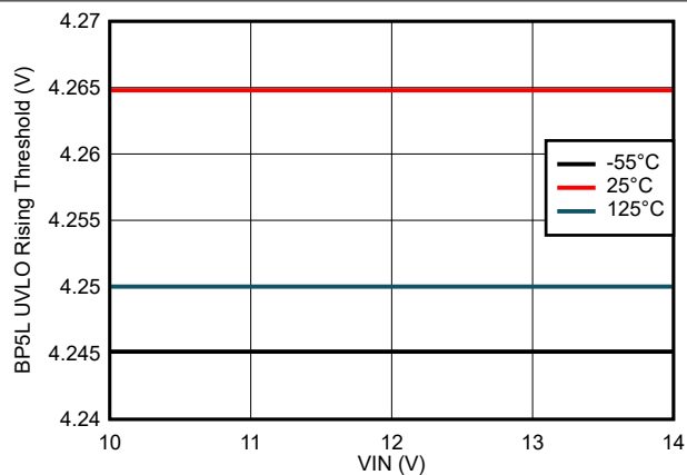
图 7-20. BP5L UVLO Rising Threshold vs VIN Voltage
