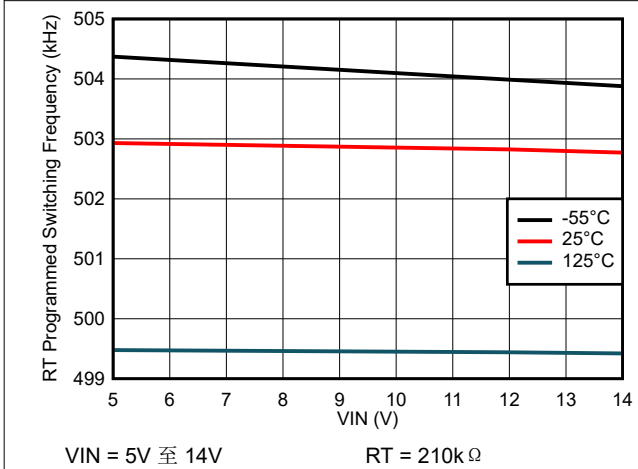
图 6-17. 开关频率与输入电压间的关系
