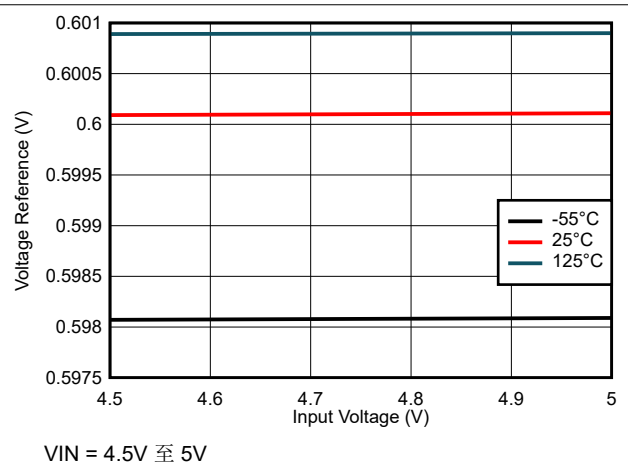
图 6-20. 内部电压基准与输入电压间的关系
