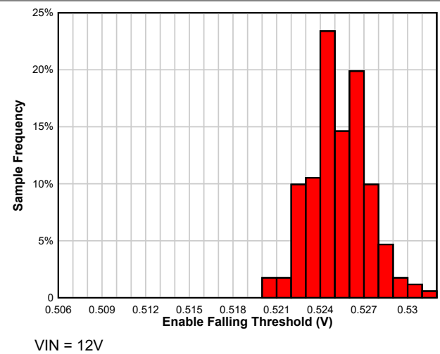
图 6-46. T_A = 125^\circ\text{C} 时的使能下降阈值分布
