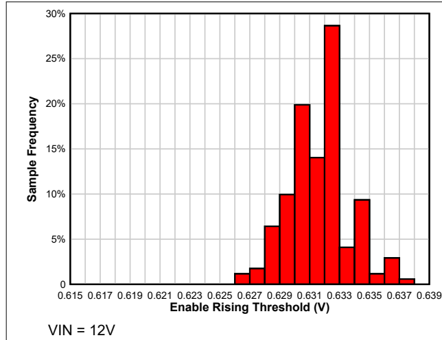
图 6-43. T_A = 125^\circ\text{C} 时的使能上升阈值分布
