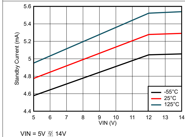
图 6-33. 待机电流与输入电压间的关系
