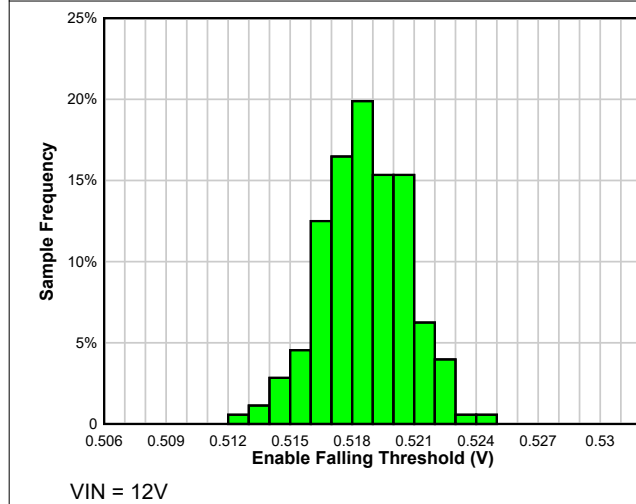
图 6-45. T_A = 25^\circ\text{C} 时的使能下降阈值分布
