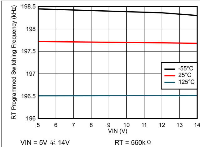
图 6-15. 开关频率与输入电压间的关系
