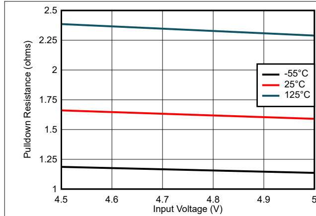
图 6-27. 下拉电阻与输入电压间的关系
