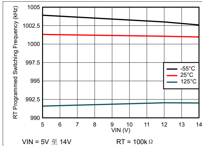
图 6-19. 开关频率与输入电压间的关系
