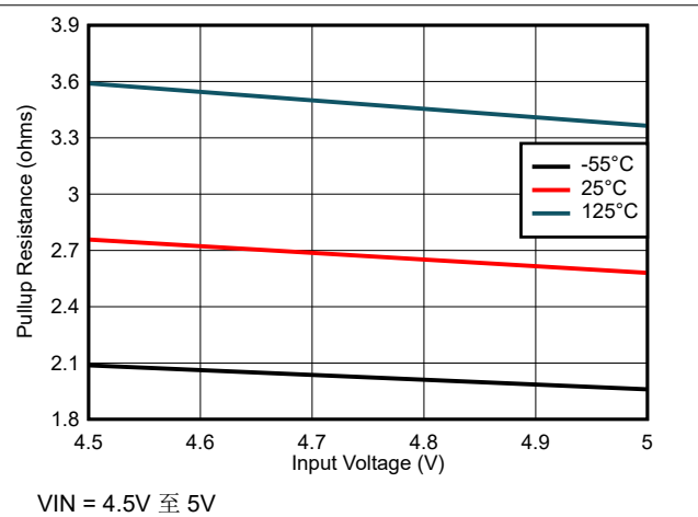
图 6-24. 上拉电阻与输入电压间的关系
