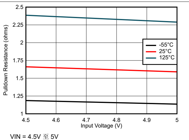
图 6-26. 下拉电阻与输入电压间的关系
