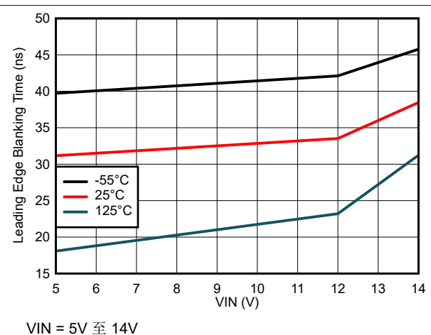
图 6-38. 前沿消隐时间与输入电压间的关系
