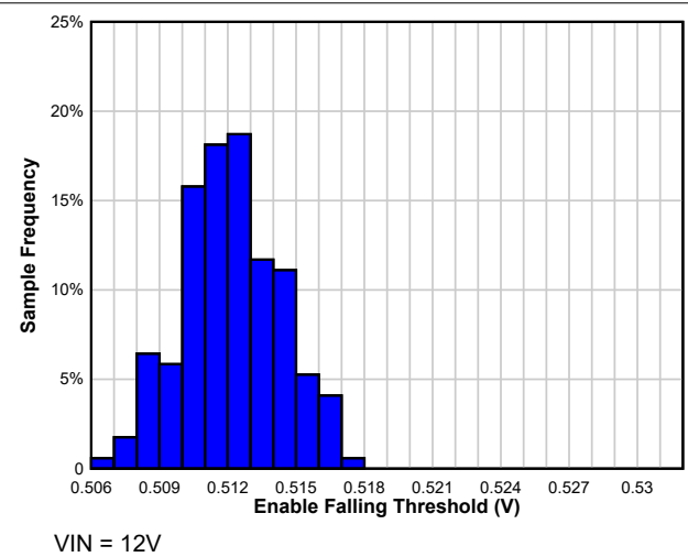
图 6-44. T_A = -55^\circ\text{C} 时的使能下降阈值分布
