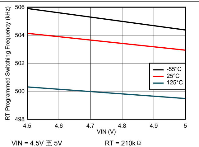
图 6-16. 开关频率与输入电压间的关系
