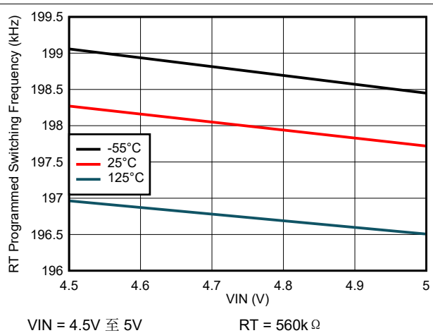
图 6-14. 开关频率与输入电压间的关系
