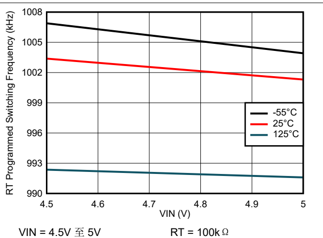
图 6-18. 开关频率与输入电压间的关系
