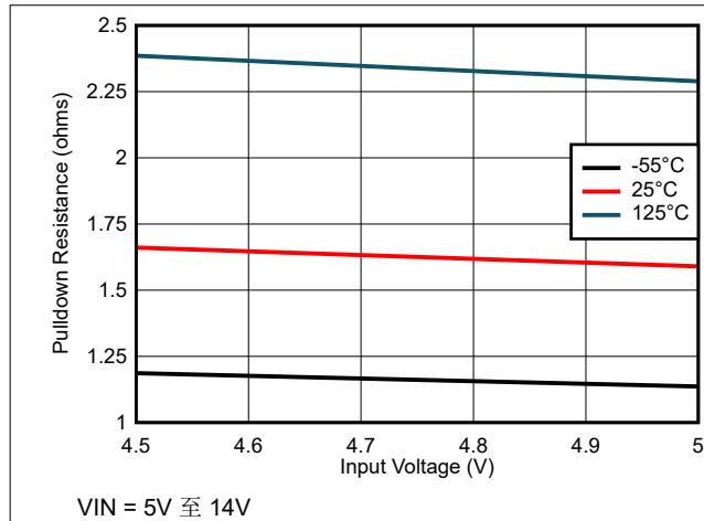
图 6-27. 下拉电阻与输入电压间的关系
